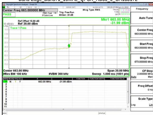
Band Edge Band71 10MHz QPSK RB50 0 CH133172
