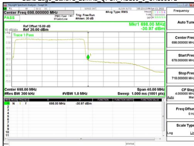
Band Edge Band71 20MHz QPSK RB100 0 CH133372
