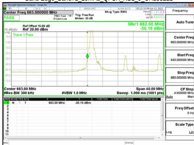
Band Edge Band71 20MHz QPSK RB1 0 CH133222
