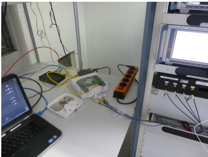
Photo 2 EUT setup
