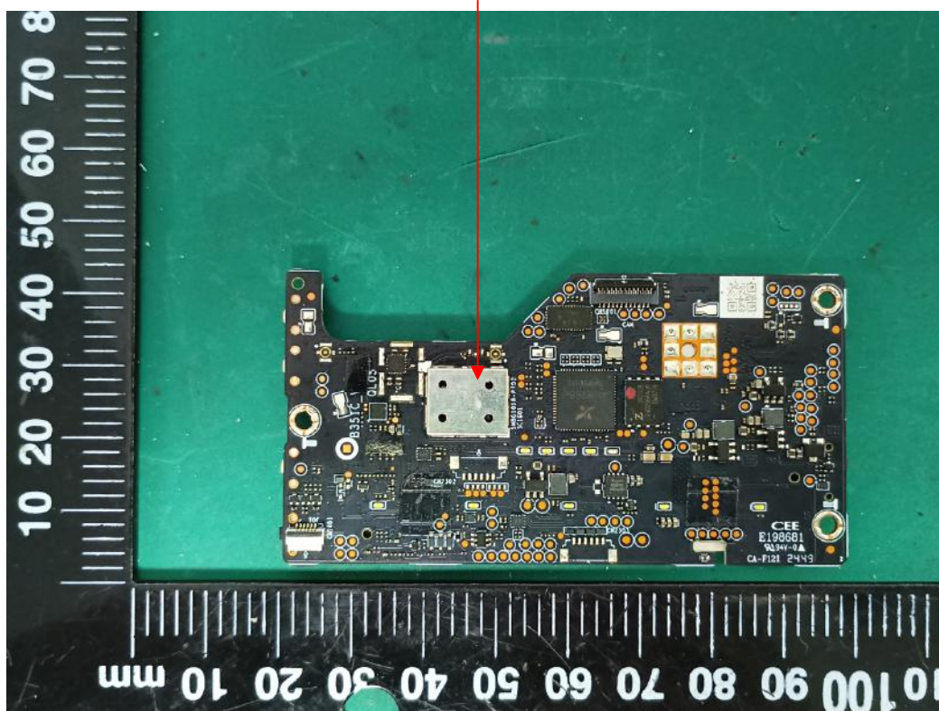
BT Module
