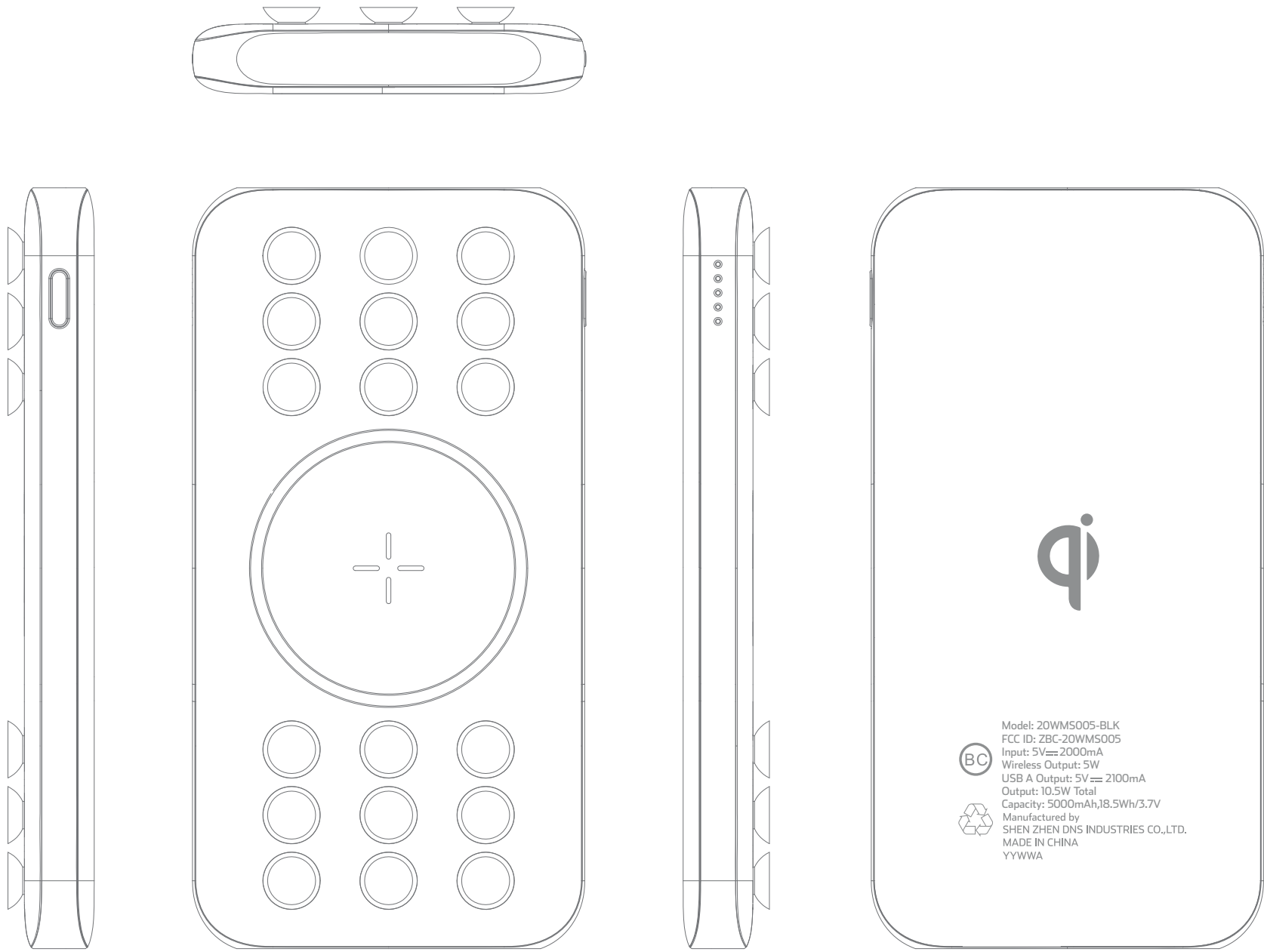
镭雕尺寸：60.6*40MM YYWWA 是Date code，格式为年年周周A，每单不同，由业务提供
