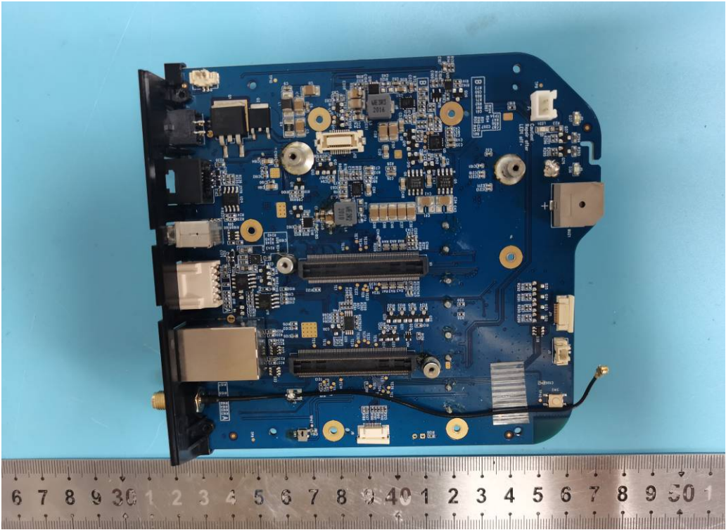
GNSS Port
