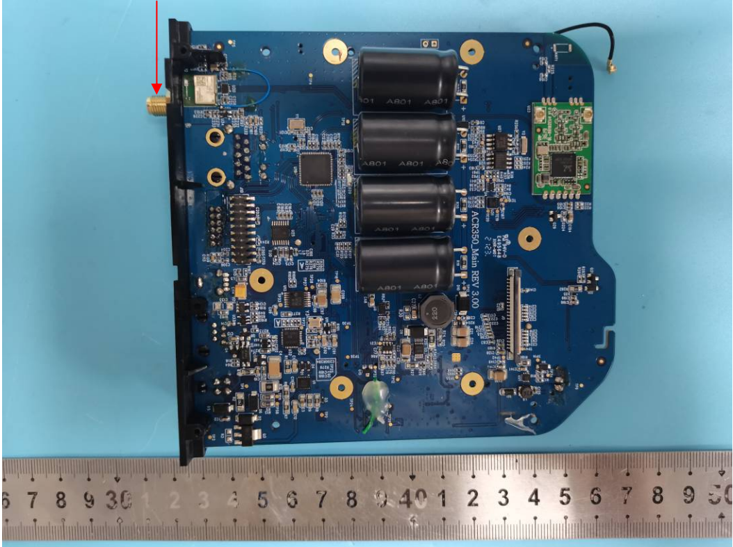
GNSS Port
