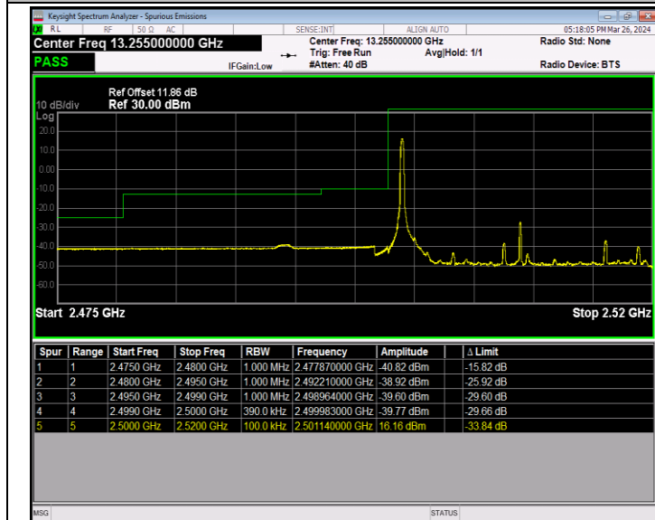
Band7_20MHz_64QAM_20850_1RB#0
