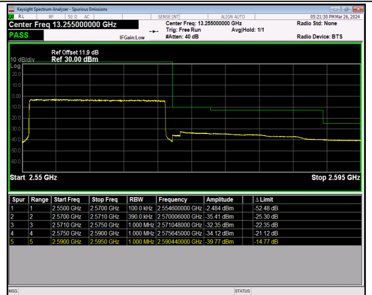
Band7_20MHz_QPSK_21350_100RB#0
