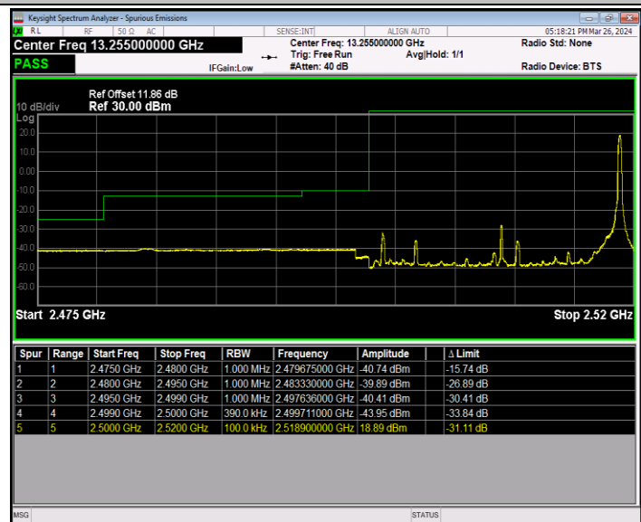
Band7_20MHz_QPSK_20850_1RB#99
