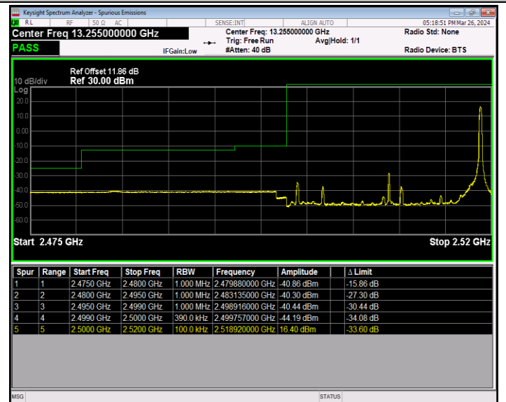
Band7_20MHz_64QAM_20850_1RB#99
