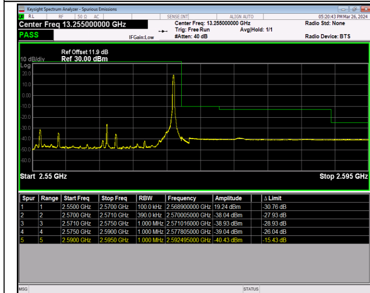
Band7_20MHz_QPSK_21350_1RB#99
