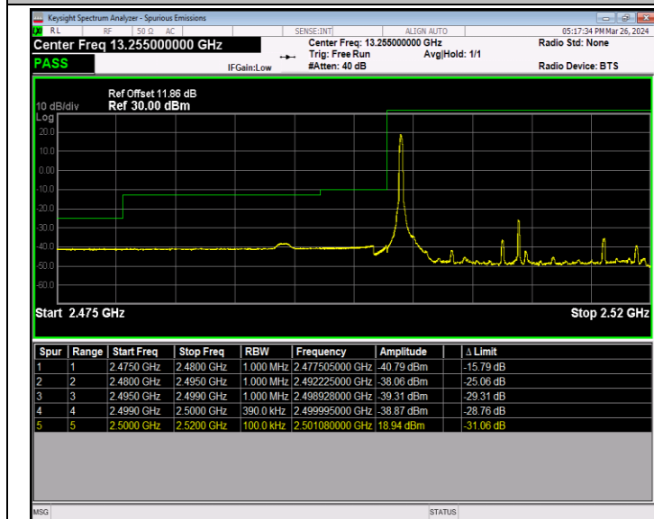
Band7_20MHz_QPSK_20850_1RB#0
