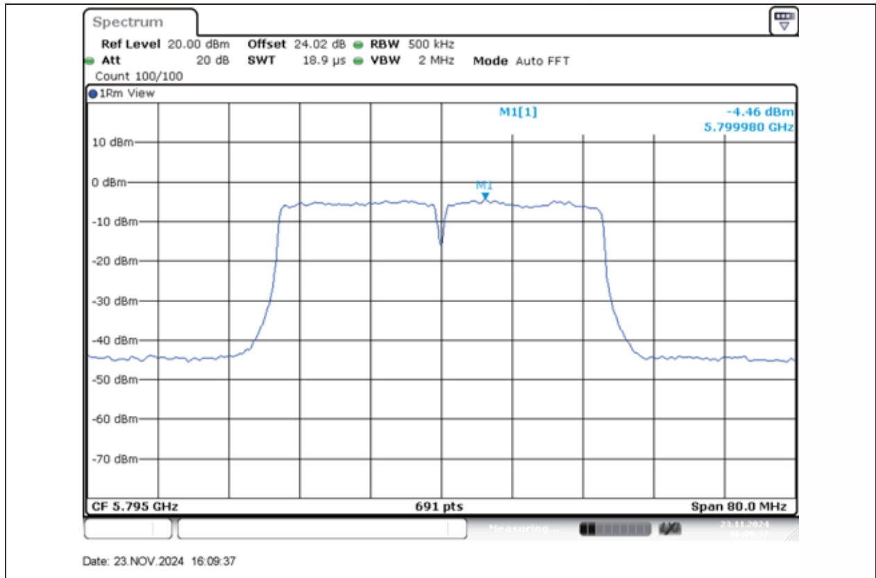
11N40MIMO-Ant1-5795-PASS
