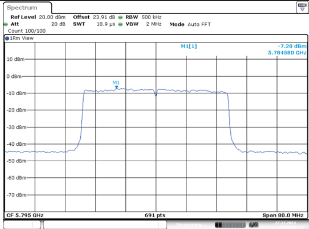
11AX40MIMO-Ant1-5795-PASS
