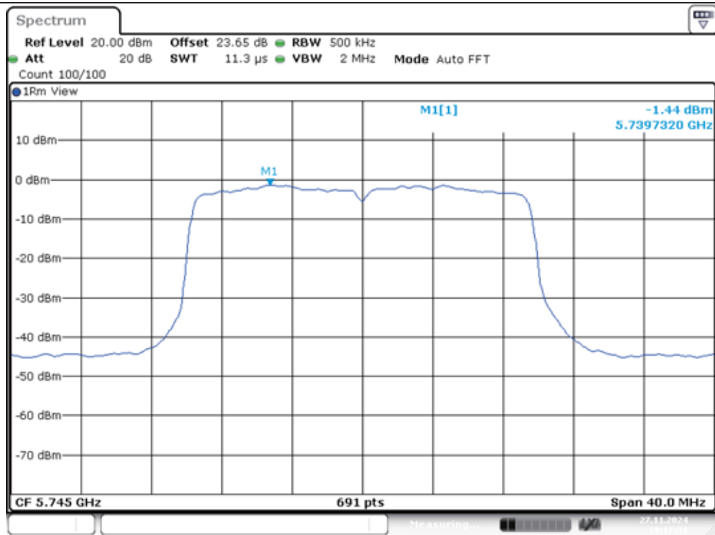
11AX20MIMO-Ant1-5745-PASS
