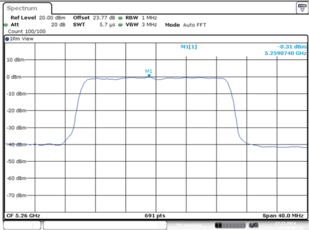
11AX20MIMO-Ant1-5260-PASS
