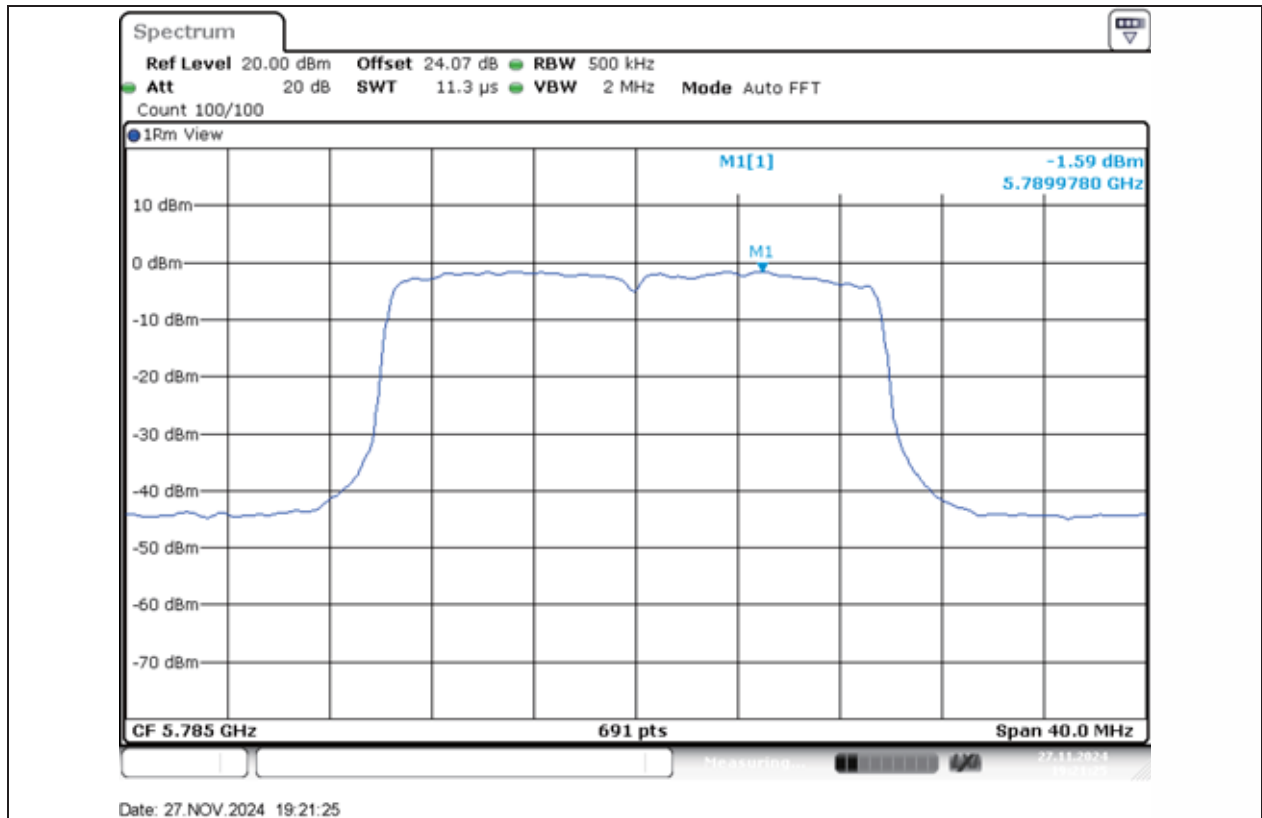
11AX20MIMO-Ant1-5785-PASS
