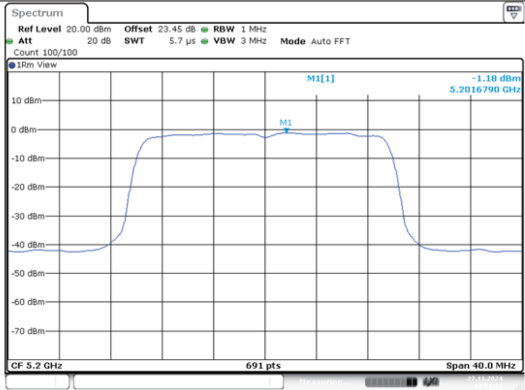
11AX20MIMO-Ant1-5200-PASS
