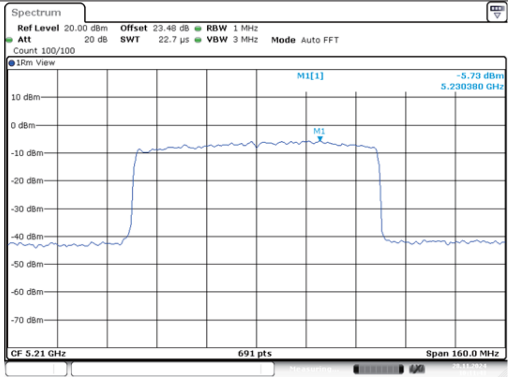
11AX80MIMO-Ant1-5210-PASS
