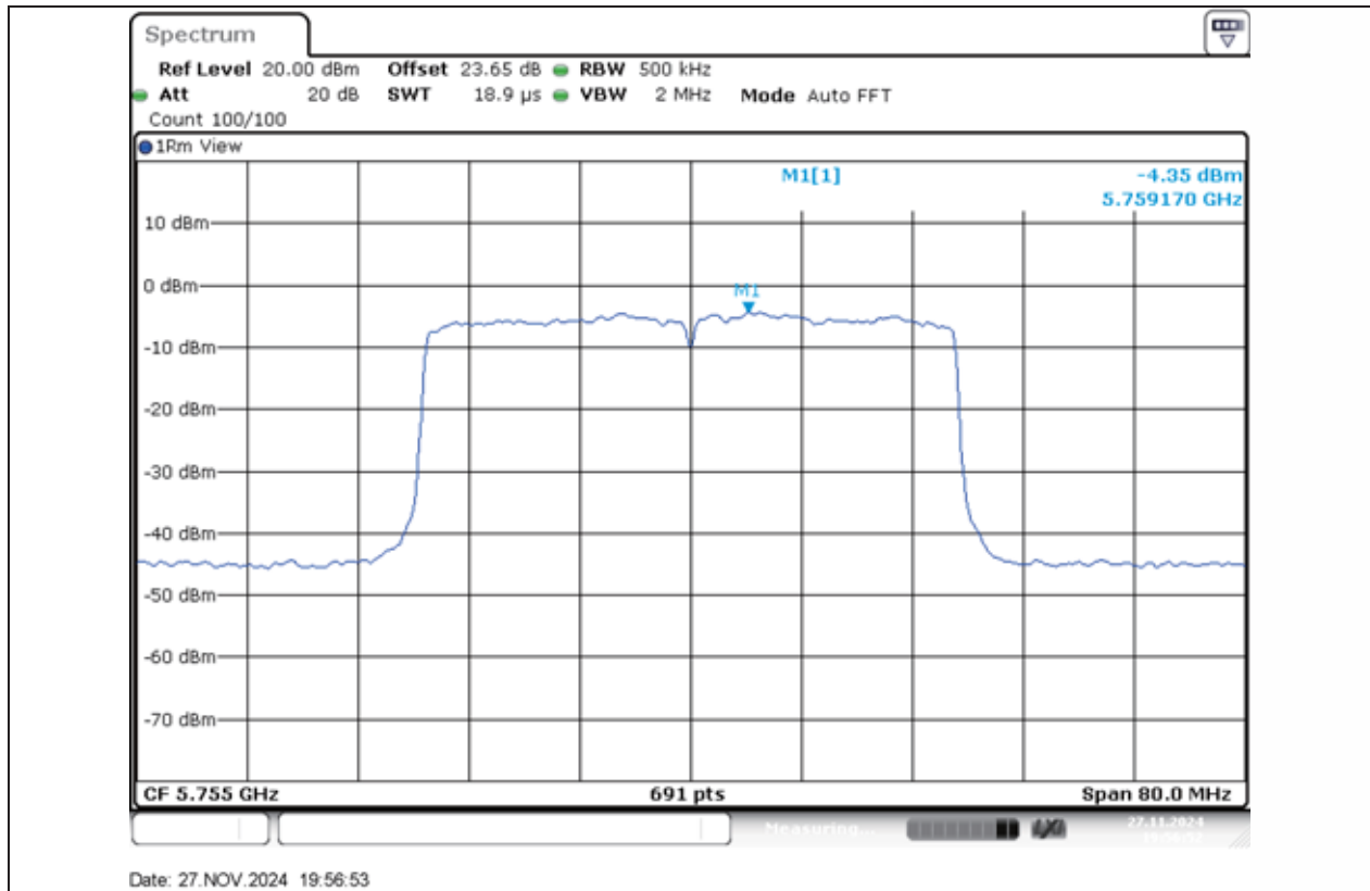
11AX40MIMO-Ant1-5755-PASS
