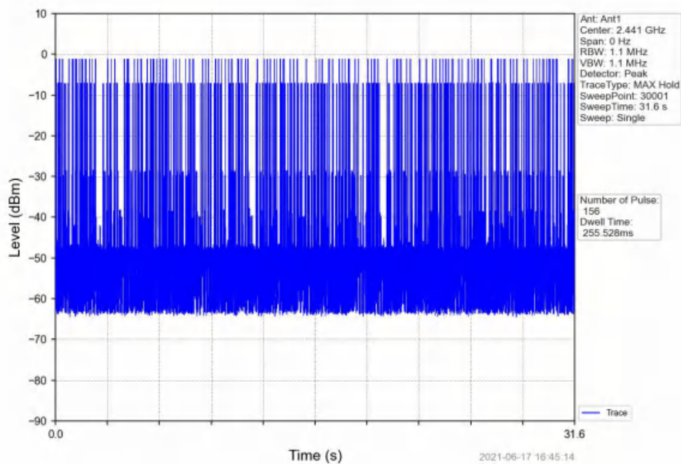
8DPSK_3DH3_HOPP_Ant1_NTNV
