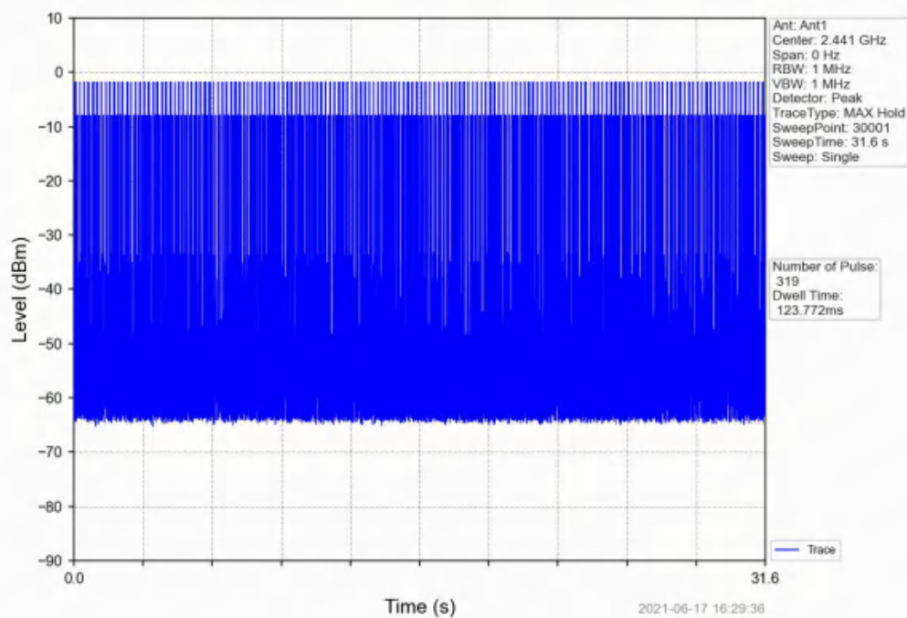
\pi/4 -DQPSK_2DH1_HOPP_Ant1_NTNV
