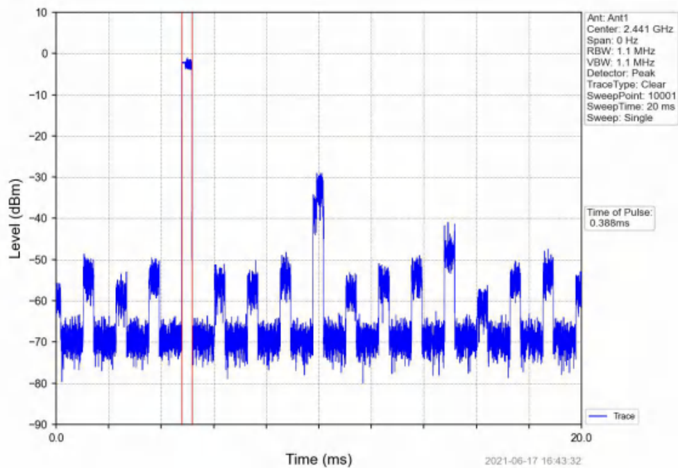
8DPSK_3DH1_HOPP_Ant1_NTNV
