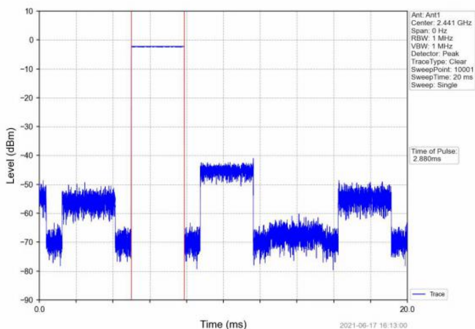
GFSK DH5_HOPP_Ant1_NTNV
