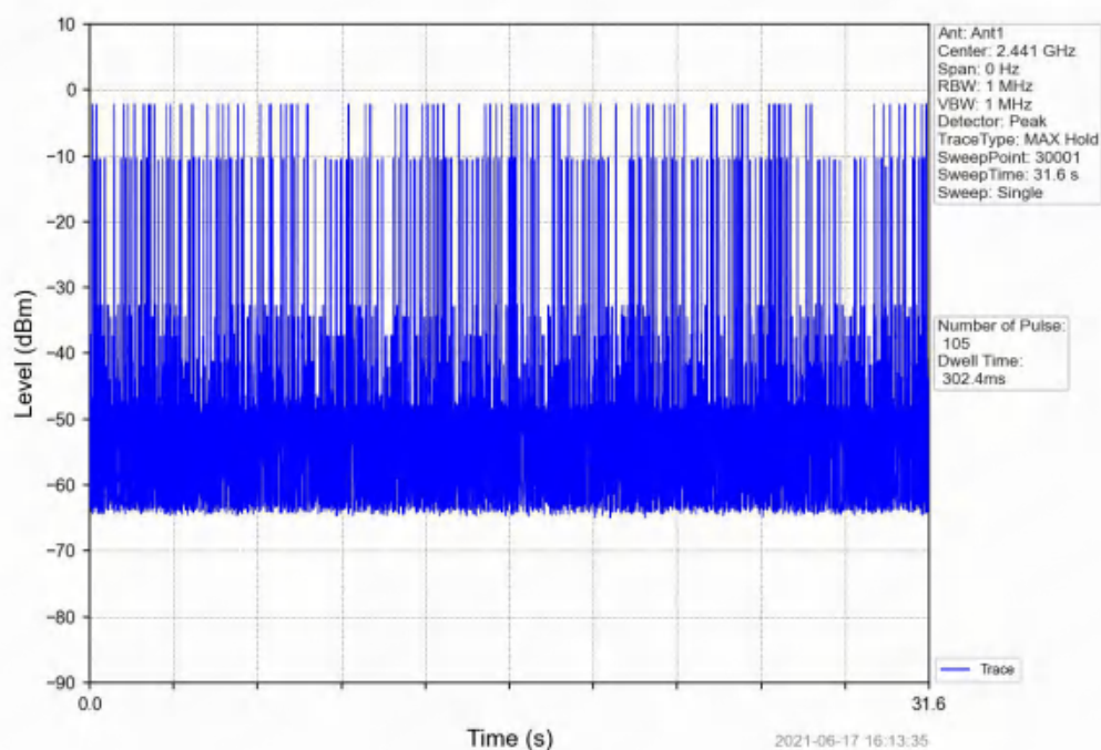
GFSK DH5_HOPP_Ant1_NTNV
