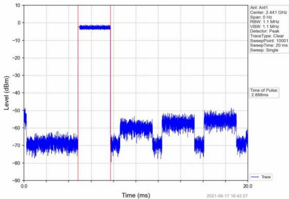
8DPSK_3DH5_HOPP_Ant1_NTNV
