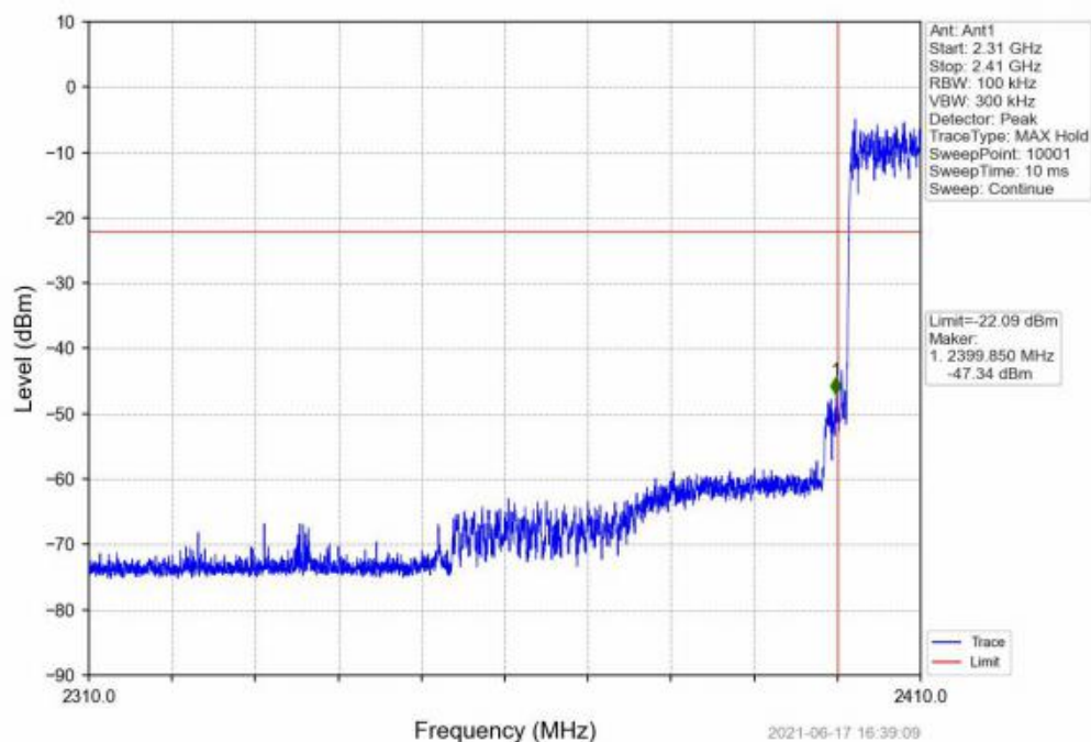
8DPSK_3DH5_HOPP_Ant1_NTNV
