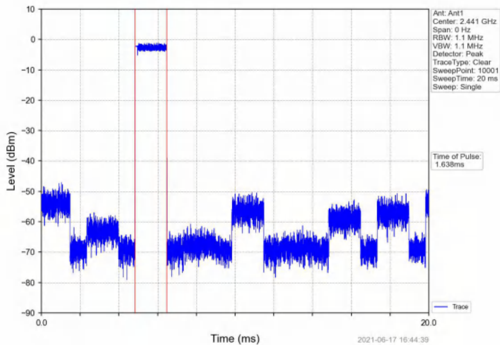
8DPSK_3DH3_HOPP_Ant1_NTNV
