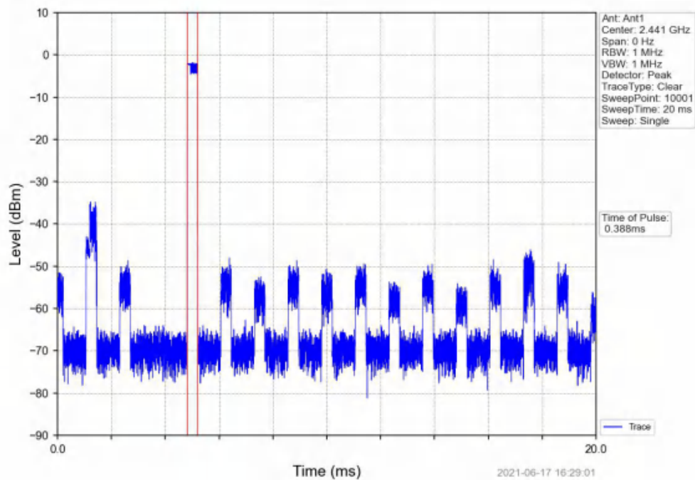
\pi/4 -DQPSK_2DH1_HOPP_Ant1_NTNV
