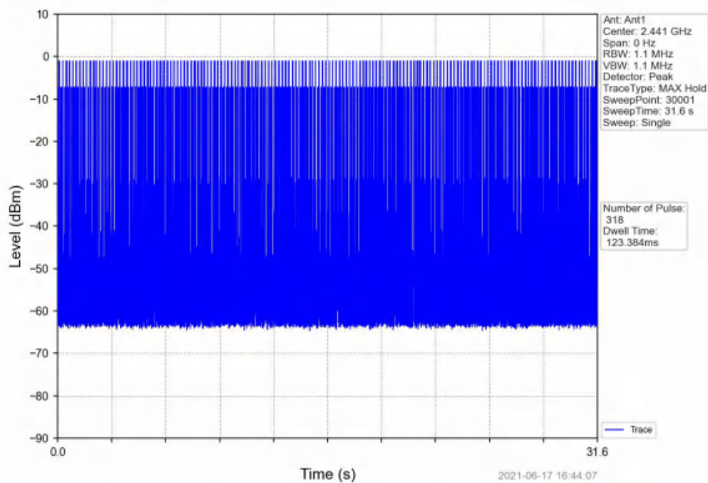
8DPSK_3DH1_HOPP_Ant1_NTNV
