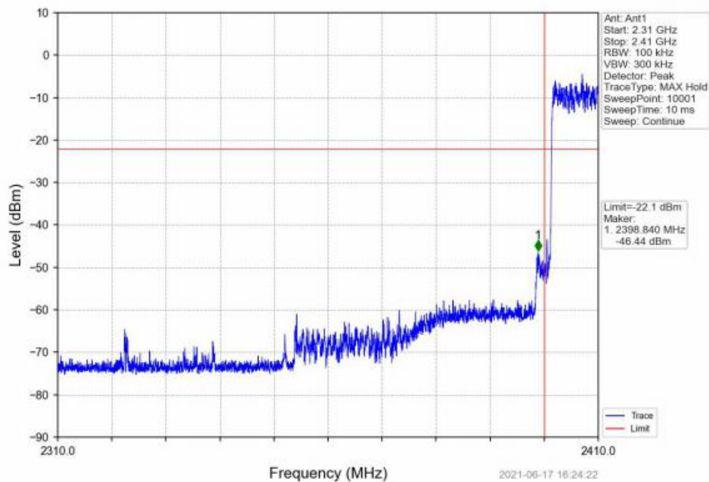
\pi /4-DQPSK_2DH5_HOPP_Ant1_NTNV
