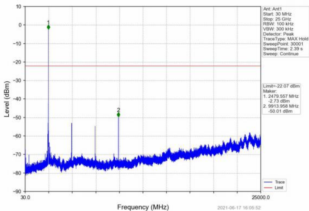
GFSK_DH5_HOPP_Ant1_NTNV
