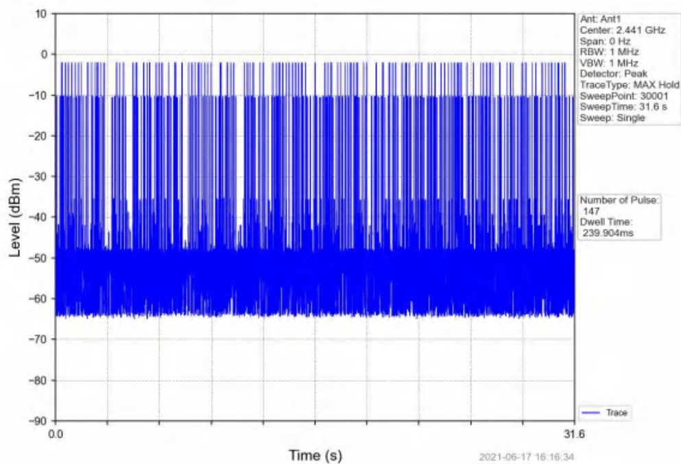
GFSK DH3_HOPP_Ant1_NTNV
