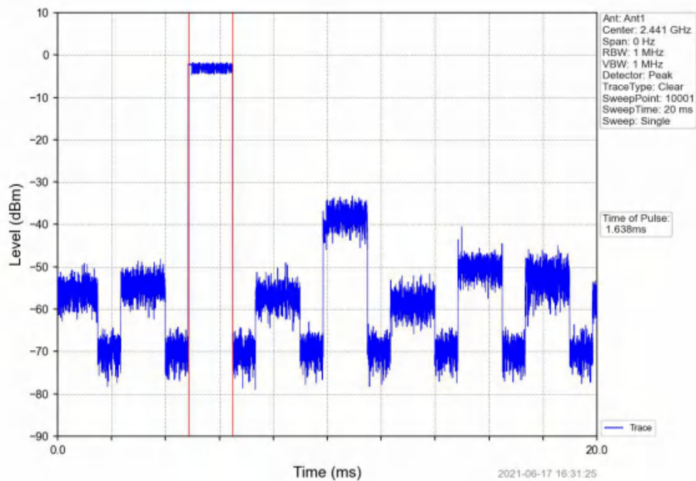
\pi /4-DQPSK_2DH3_HOPP_Ant1_NTNV
