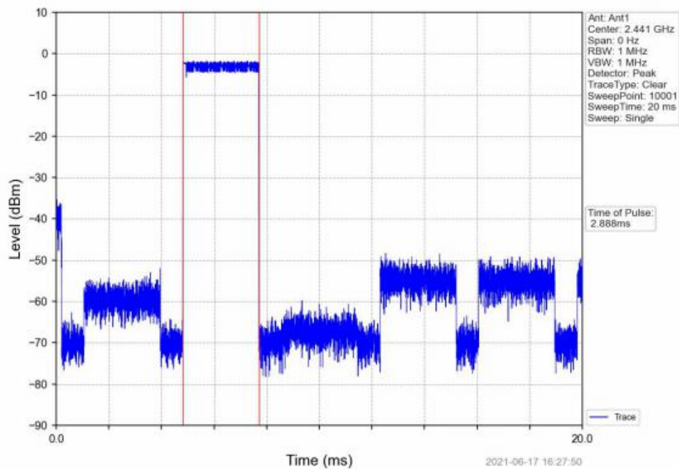
\pi /4-DQPSK_2DH5_HOPP_Ant1_NTNV
