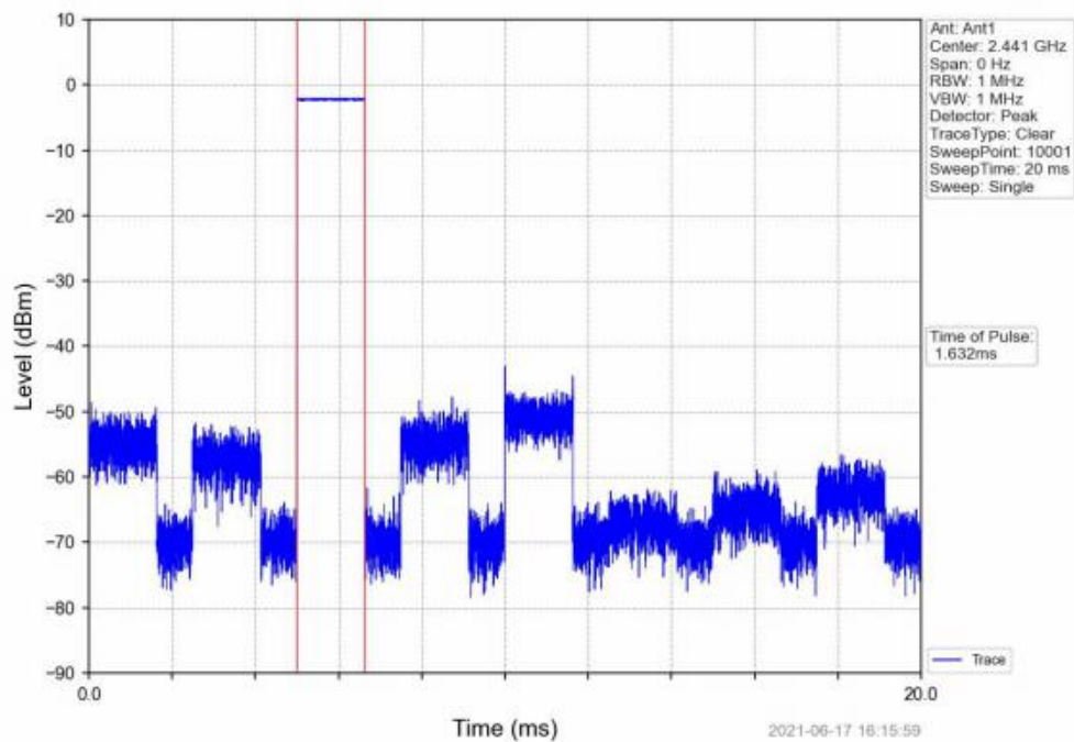
GFSK DH3_HOPP_Ant1_NTNV
