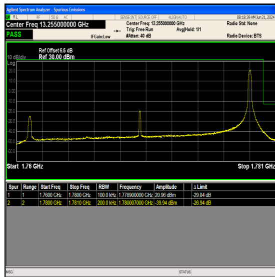
Band66_20MHz_QPSK_132572_1RB#99
