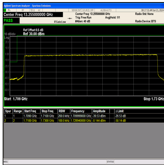
Band66_20MHz_QPSK_132072_100RB#0
