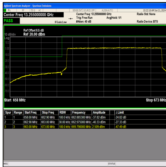
Band71_10MHz_QPSK_133172_50RB#0
