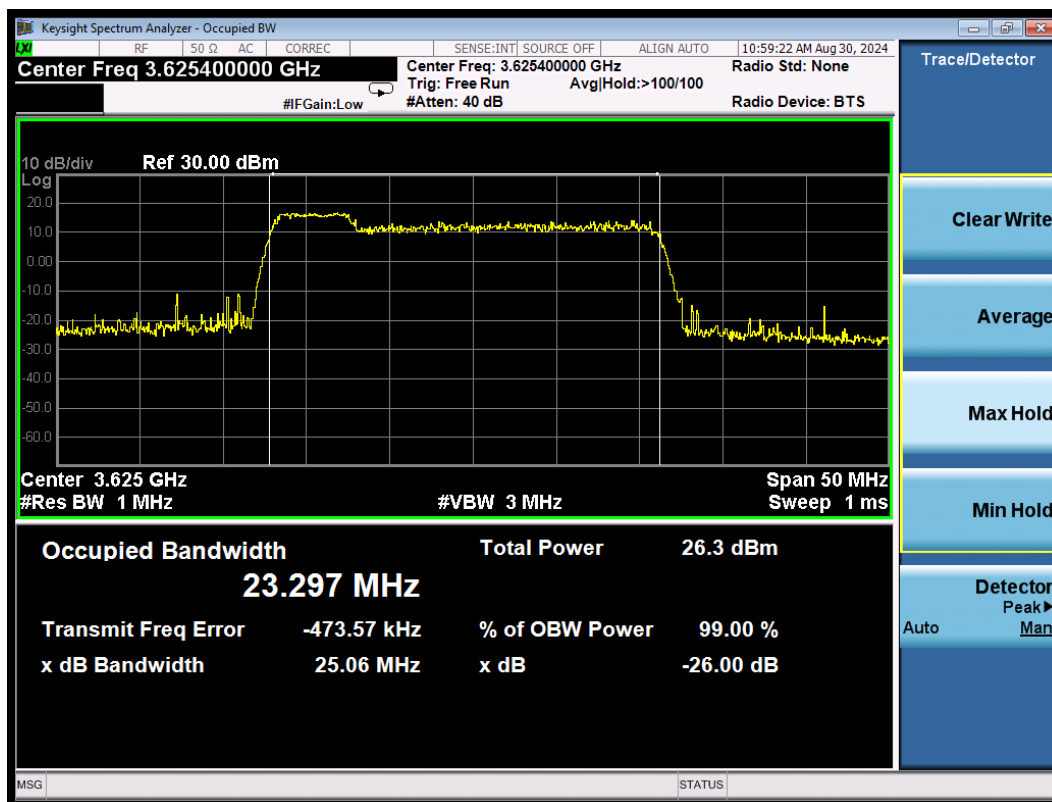
CA_48C QPSK\5MHz+20MHz Middle
