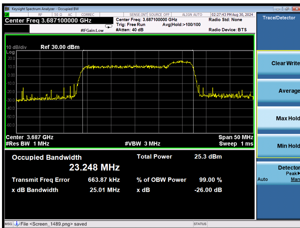
CA_48C 64QAM\20MHz+5MHz High
