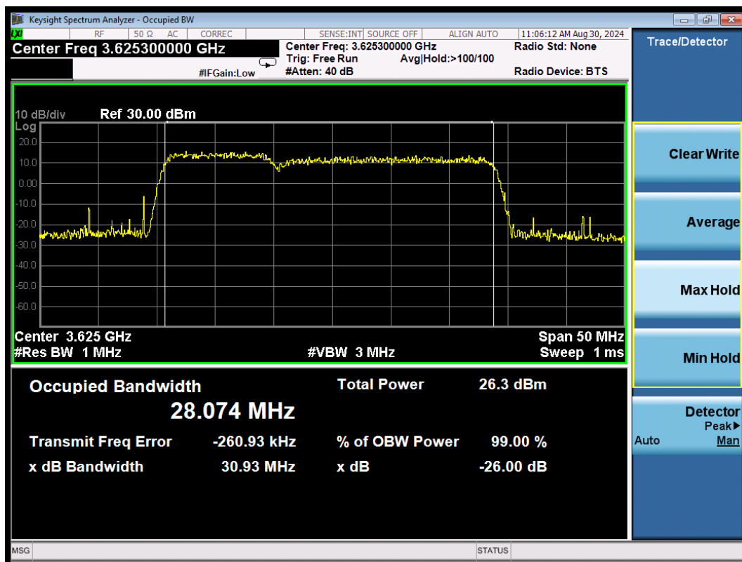
CA_48C 16QAM\10MHz+20MHz Middle
