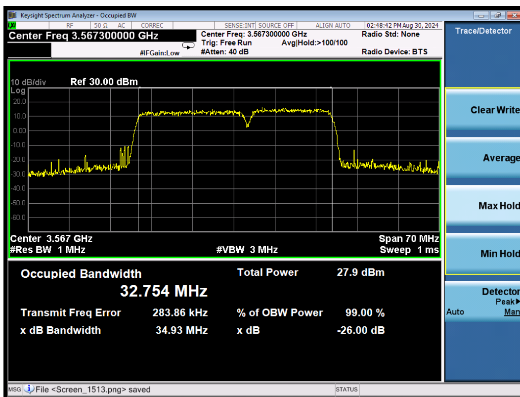
CA_48C QPSK\20MHz+15MHz Low
