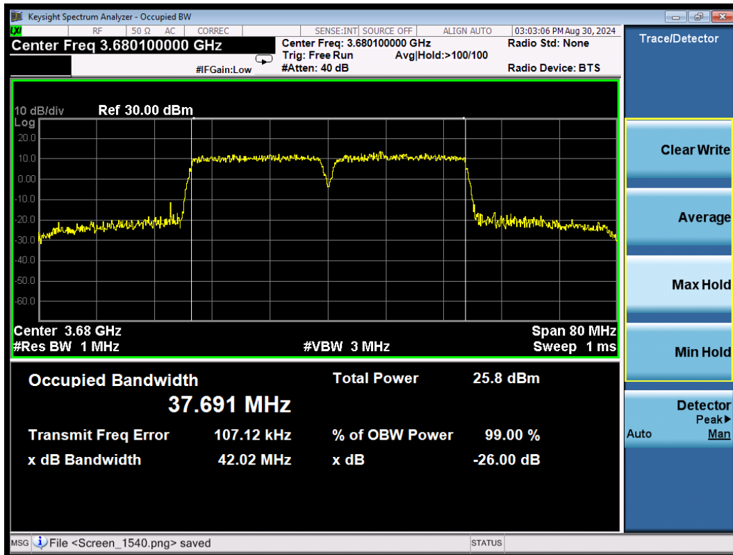
CA_48C 64QAM\20MHz+20MHz High
