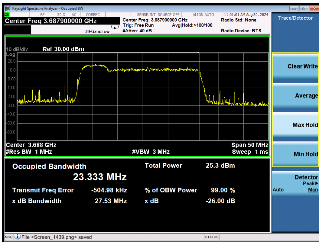
CA_48C 16QAM\5MHz+20MHz High
