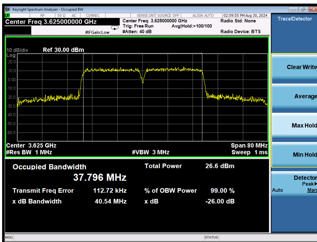
CA_48C 64QAM\20MHz+20MHz Middle
