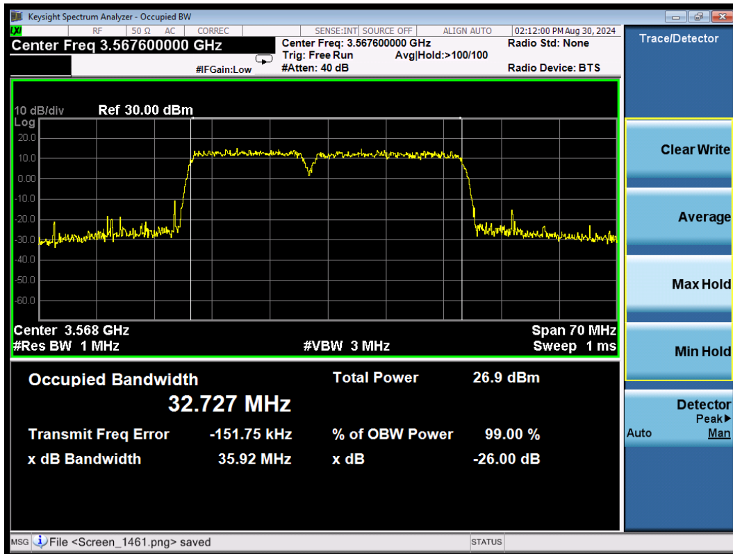
CA_48C 64QAM\15MHz+20MHz Low
