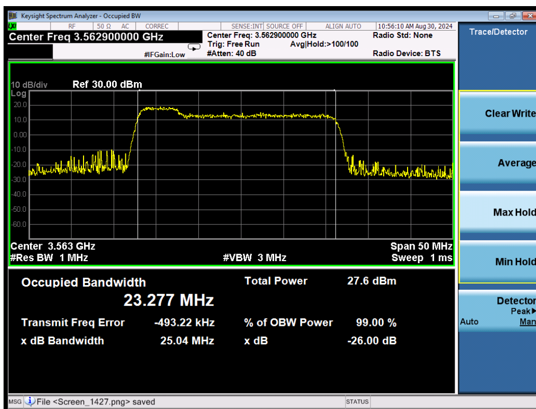
CA_48C 64QAM\5MHz+20MHz Low
