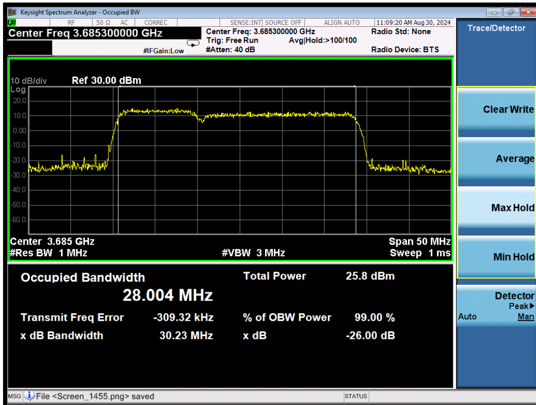
CA_48C 64QAM\10MHz+20MHz High
