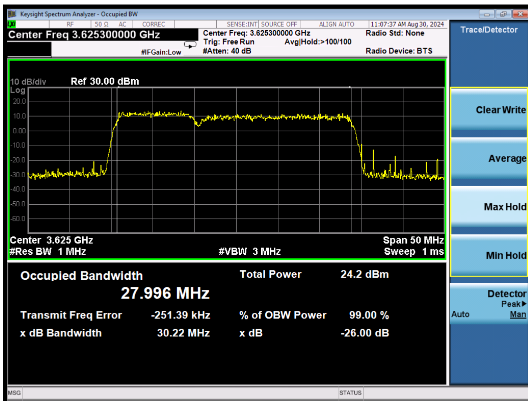
CA_48C 256QAM\10MHz+20MHz Middle
