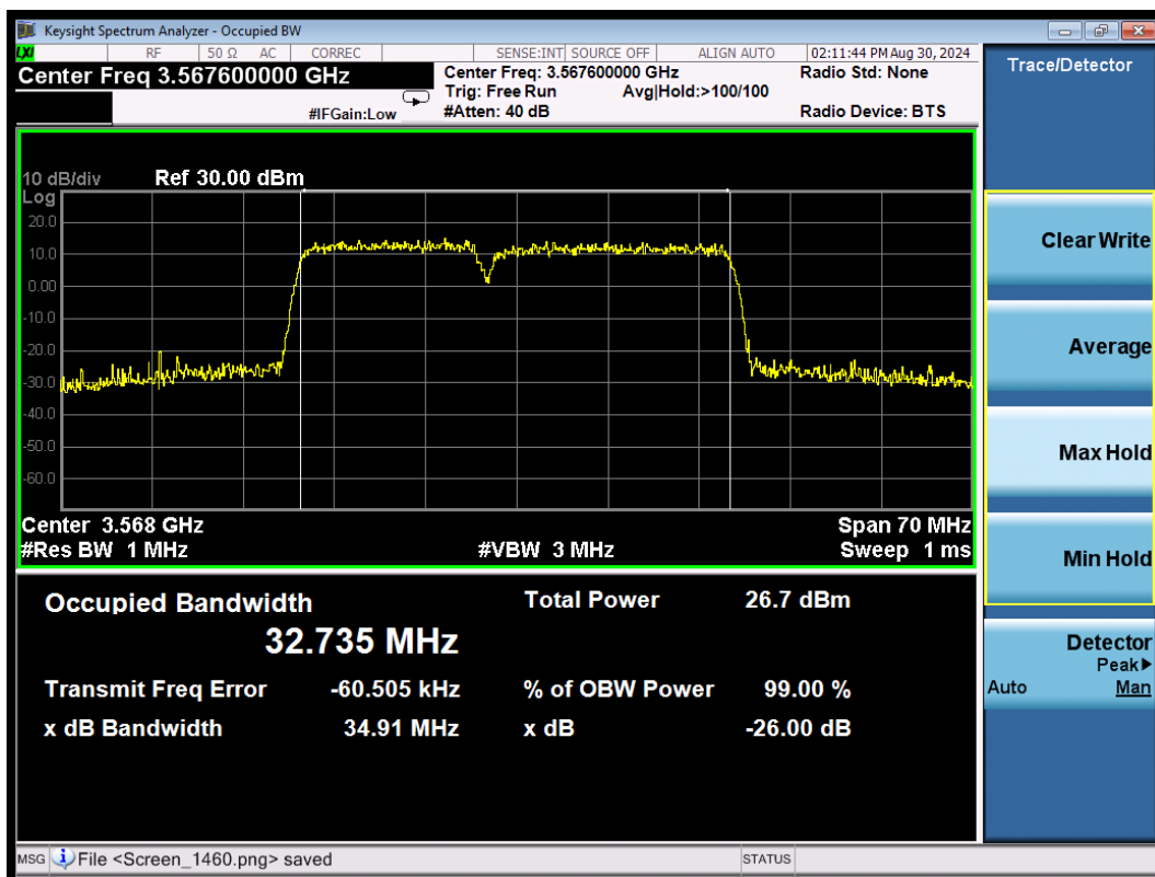
CA_48C 16QAM\15MHz+20MHz Low
