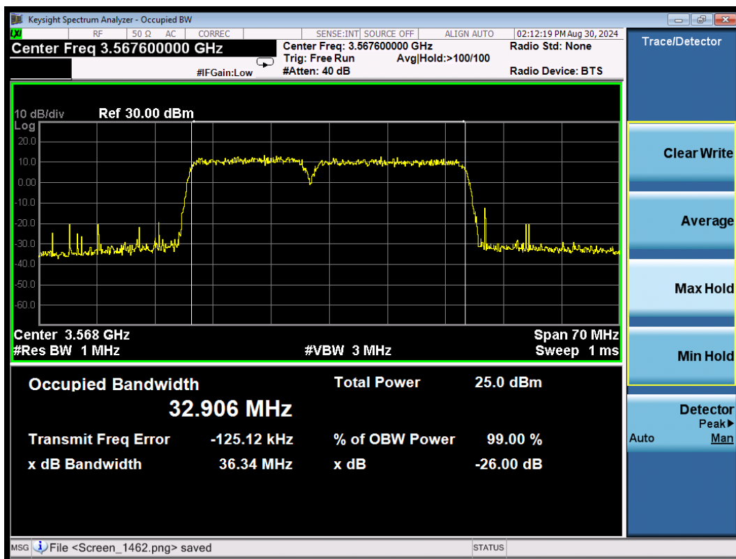
CA_48C 256QAM\15MHz+20MHz Low
