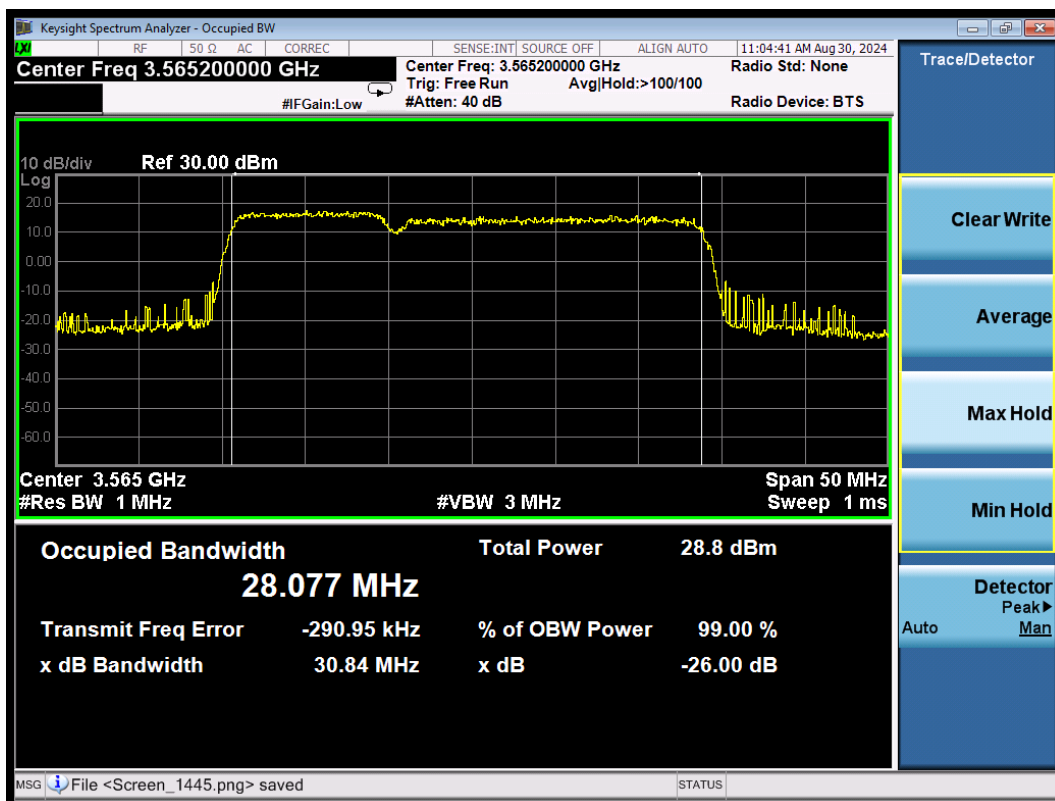
CA_48C QPSK\10MHz+20MHz Low
