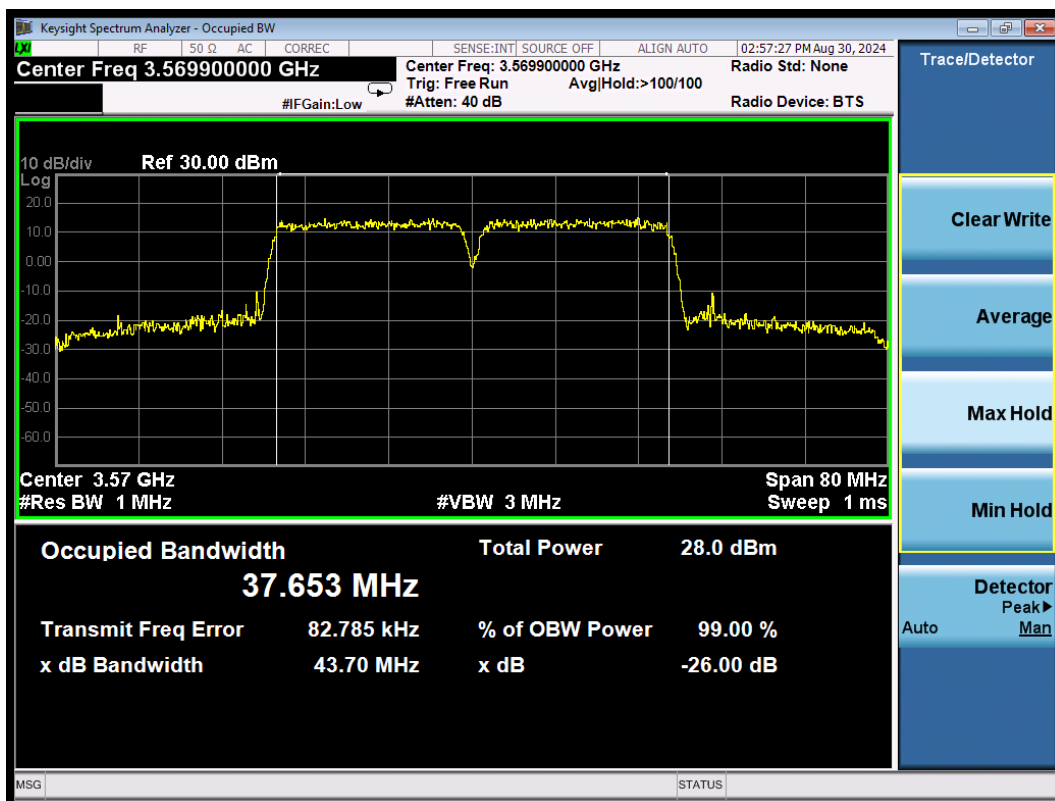
CA_48C QPSK\20MHz+20MHz Low
