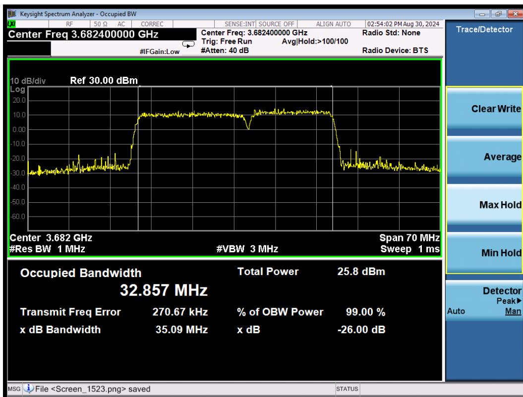
CA_48C 64QAM\20MHz+15MHz High
