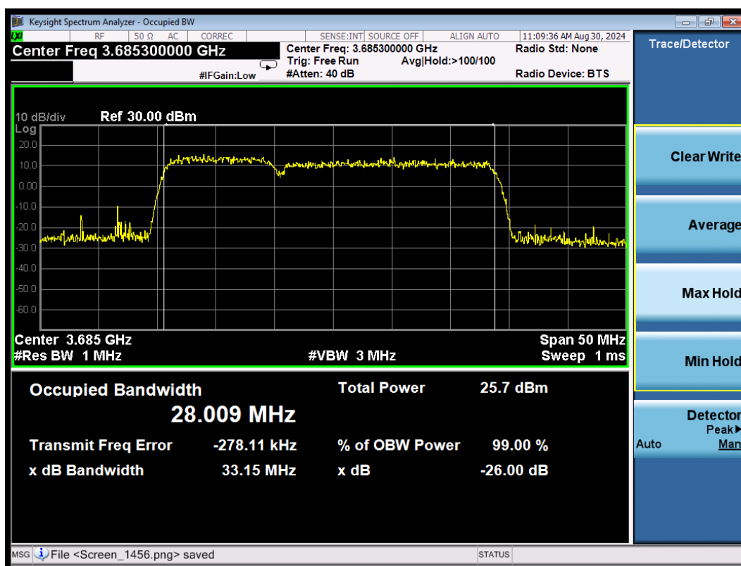
CA_48C 16QAM\10MHz+20MHz High
