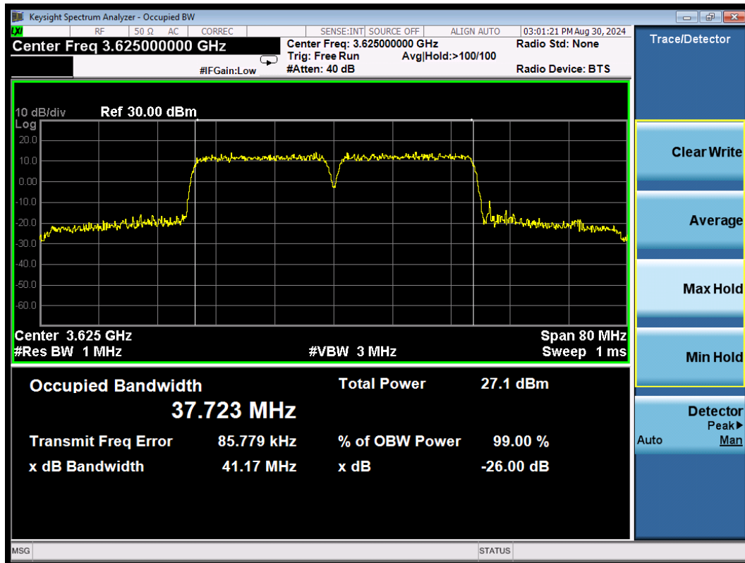
CA_48C QPSK\20MHz+20MHz Middle
