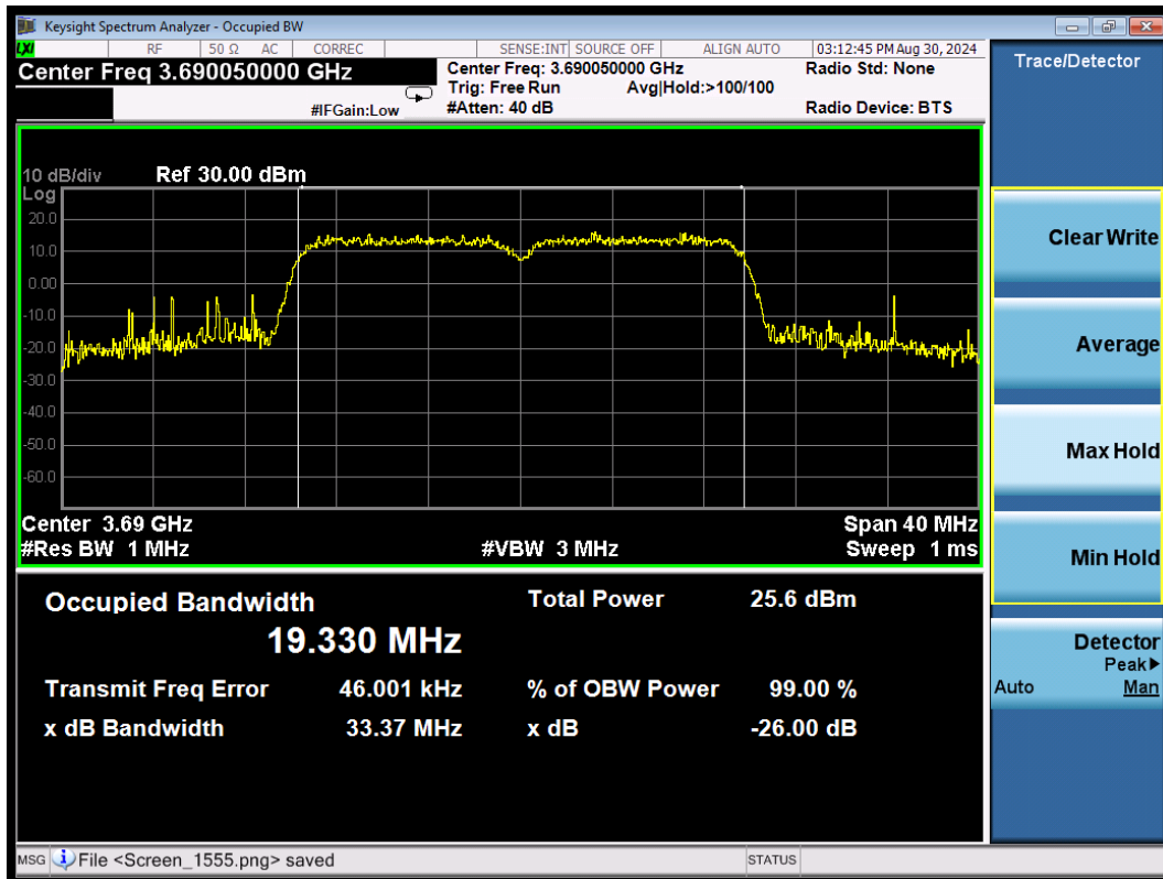
CA_48B 64QAM\10MHz+10MHz High
