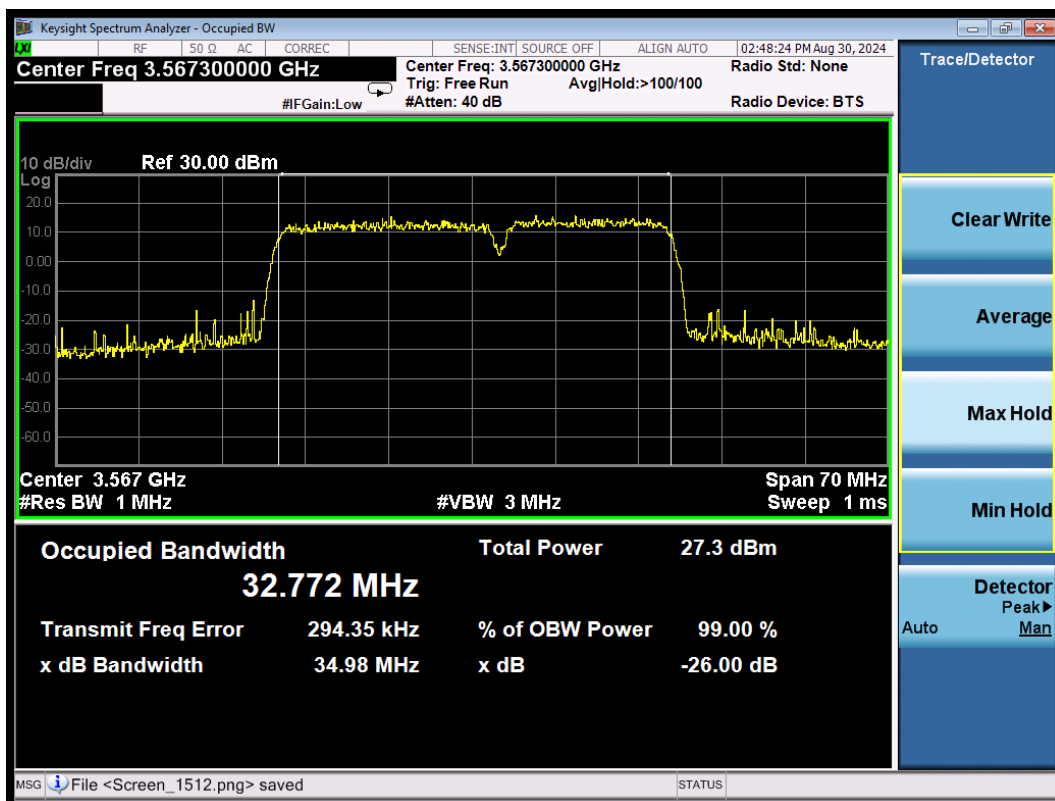
CA_48C 16QAM\20MHz+15MHz Low
