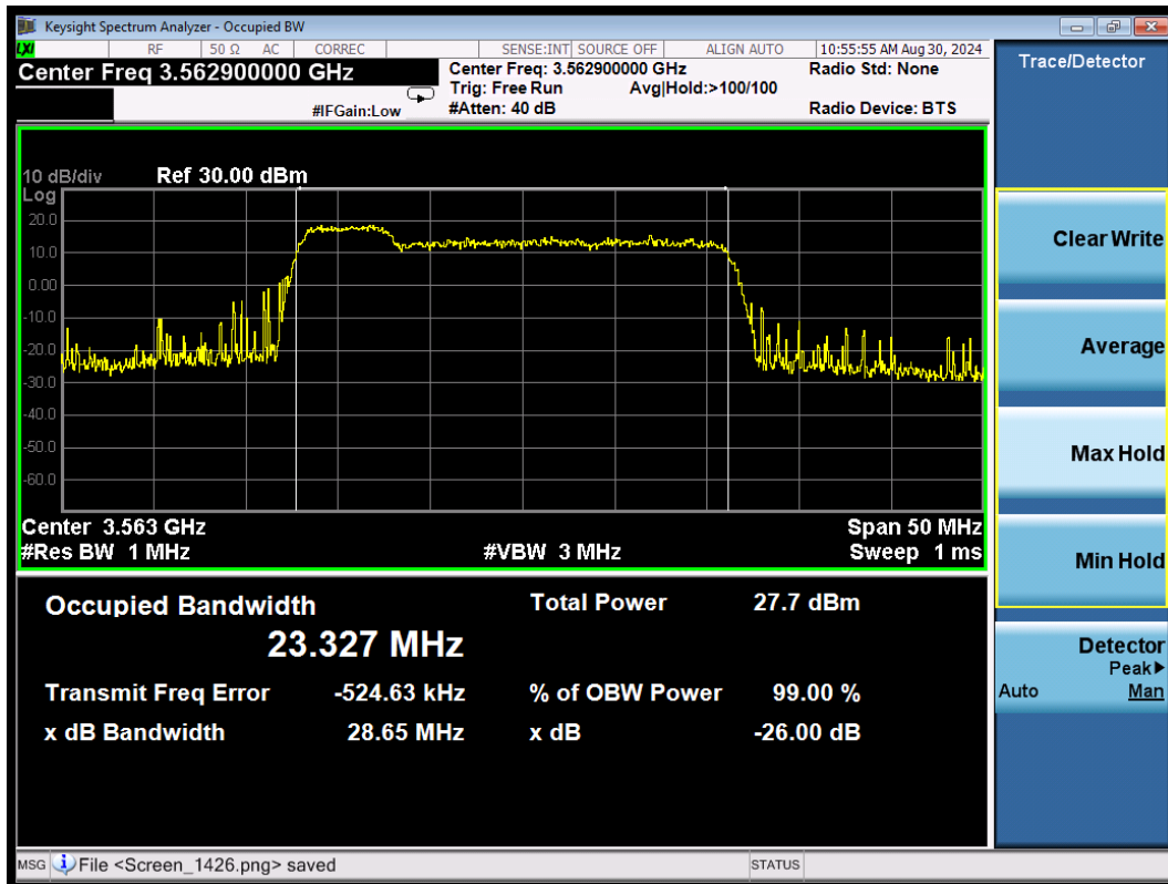
CA_48C 16QAM\5MHz+20MHz Low
