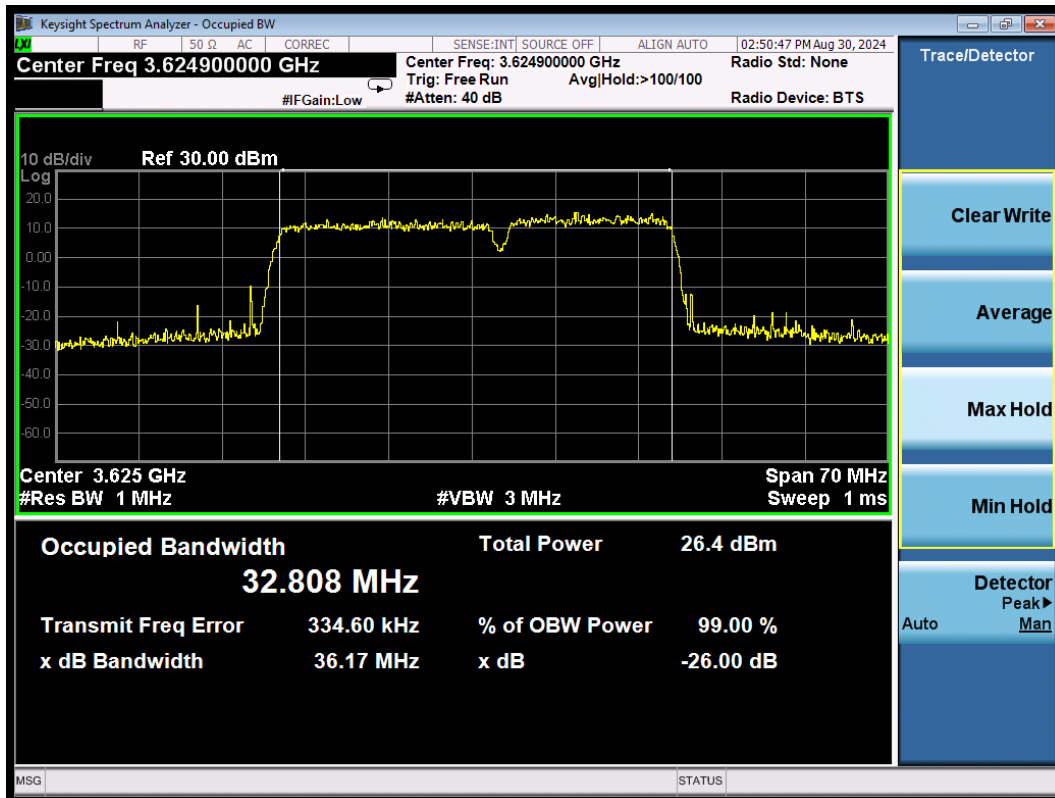
CA_48C 16QAM\20MHz+15MHz Middle
