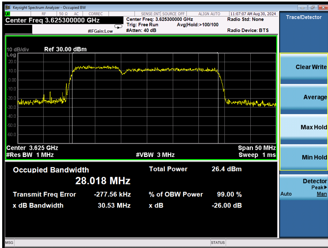
CA_48C 64QAM\10MHz+20MHz Middle
