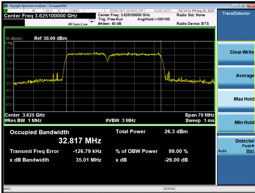
CA_48C 16QAM\15MHz+20MHz Middle
