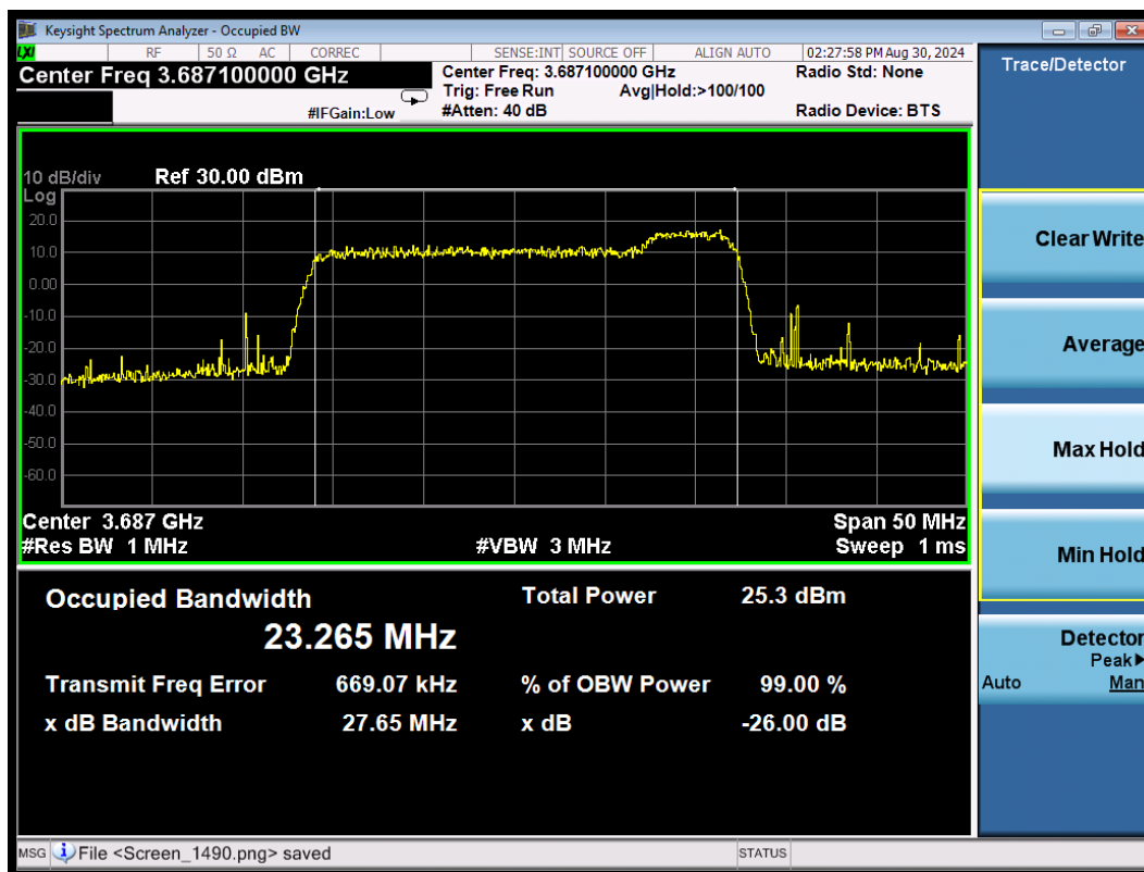
CA_48C 16QAM\20MHz+5MHz High
