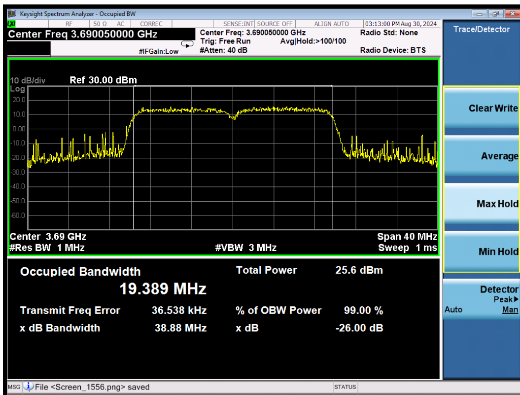
CA_48B 16QAM\10MHz+10MHz High
