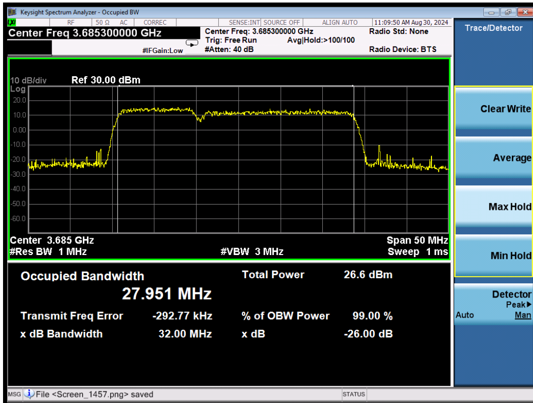
CA_48C QPSK\10MHz+20MHz High
