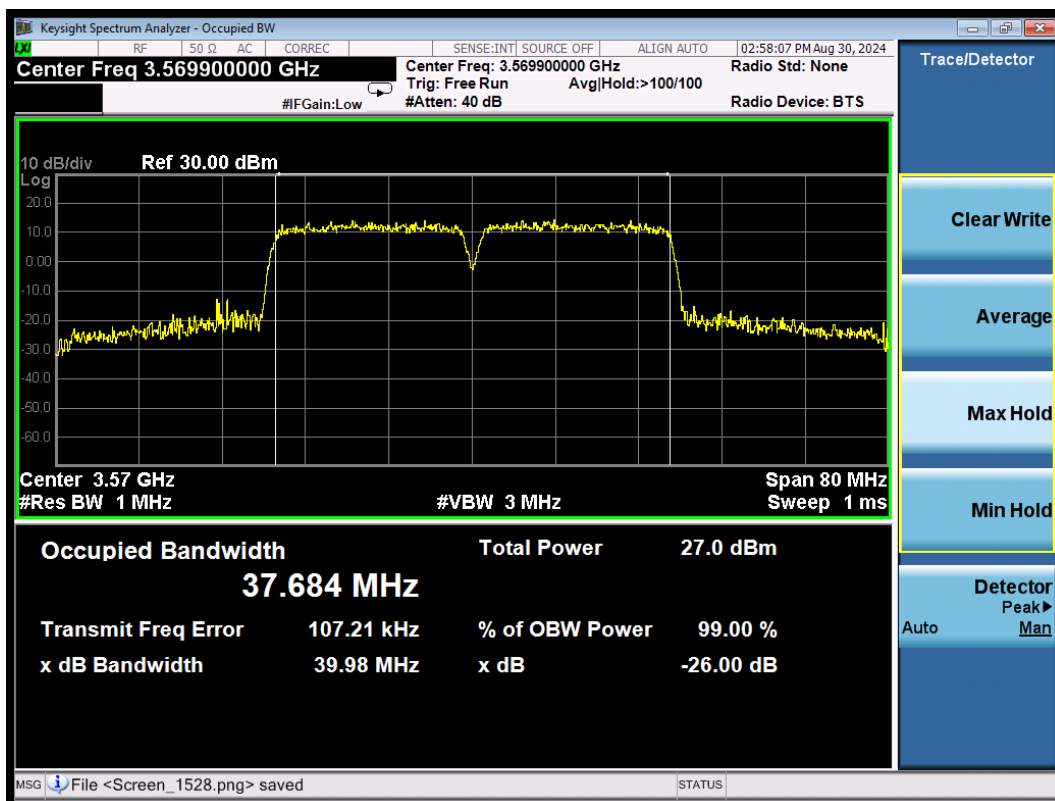
CA_48C 64QAM\20MHz+20MHz Low
