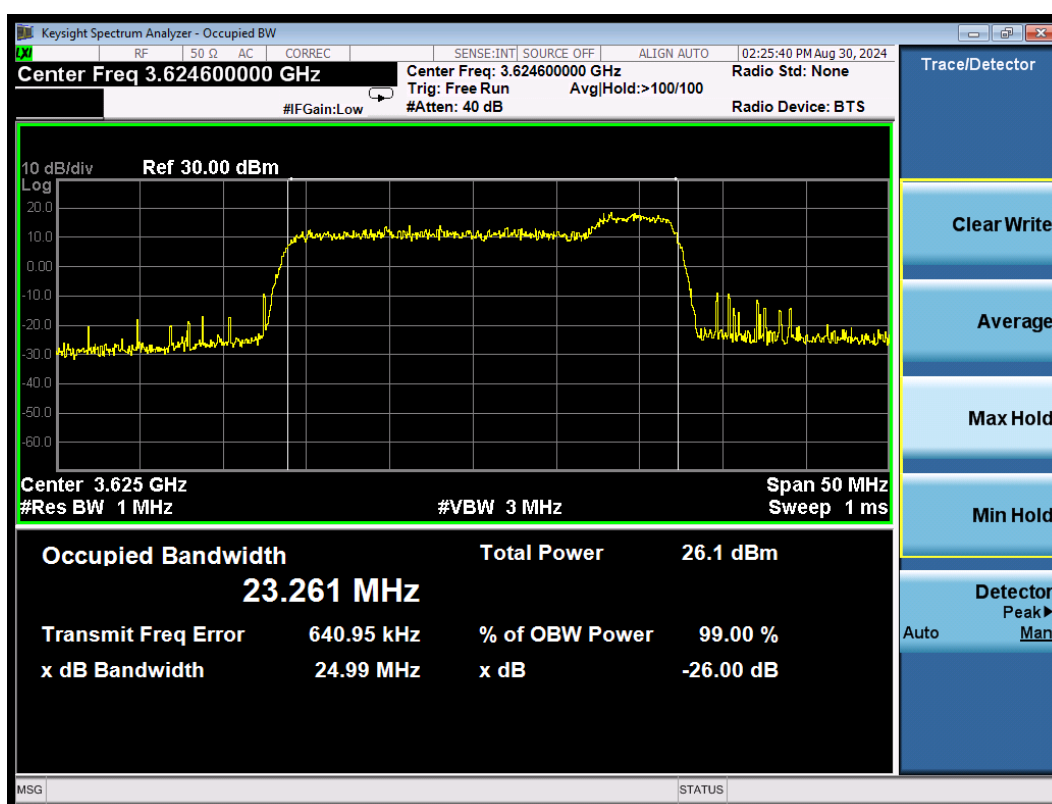
CA_48C 64QAM\20MHz+5MHz Middle
