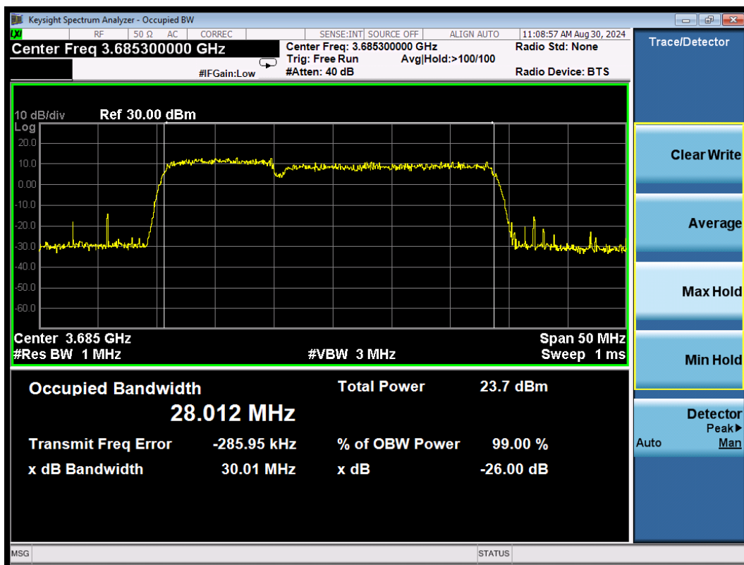
CA_48C 256QAM\10MHz+20MHz High
