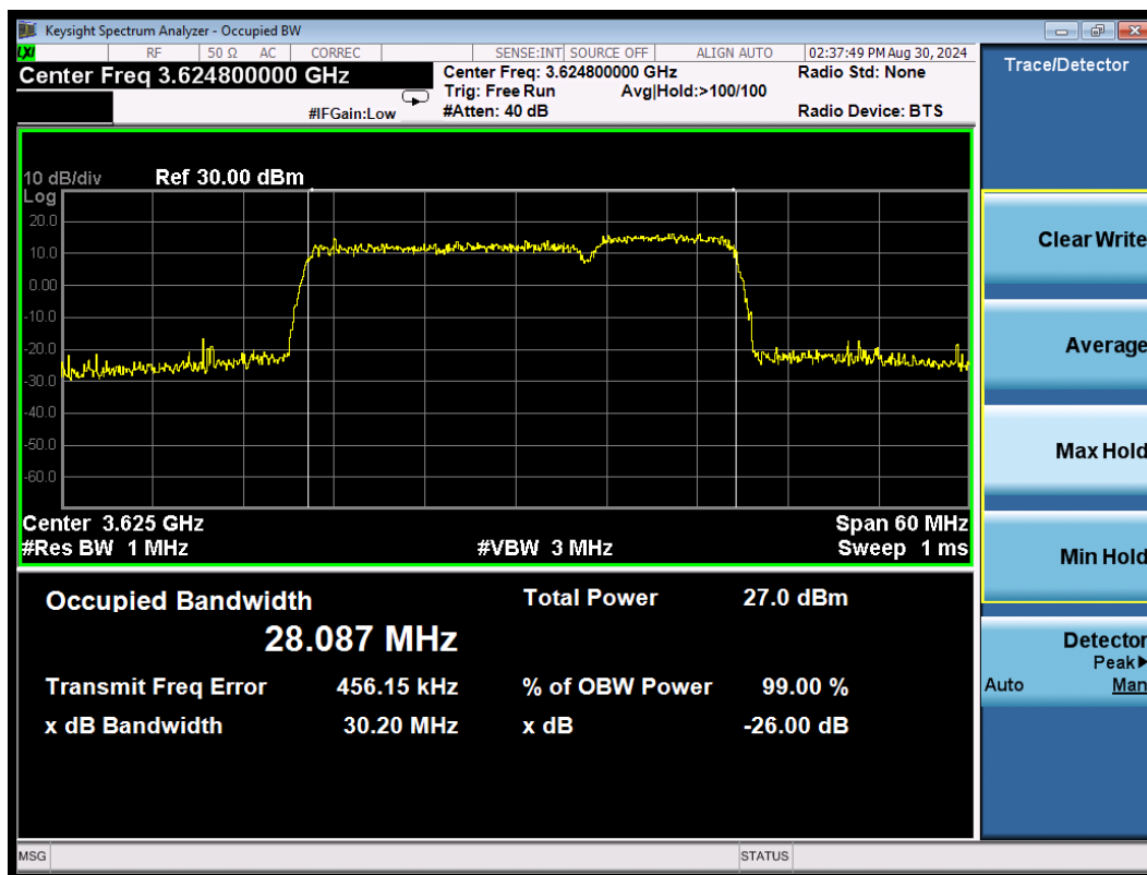
CA_48C QPSK\20MHz+10MHz Middle
