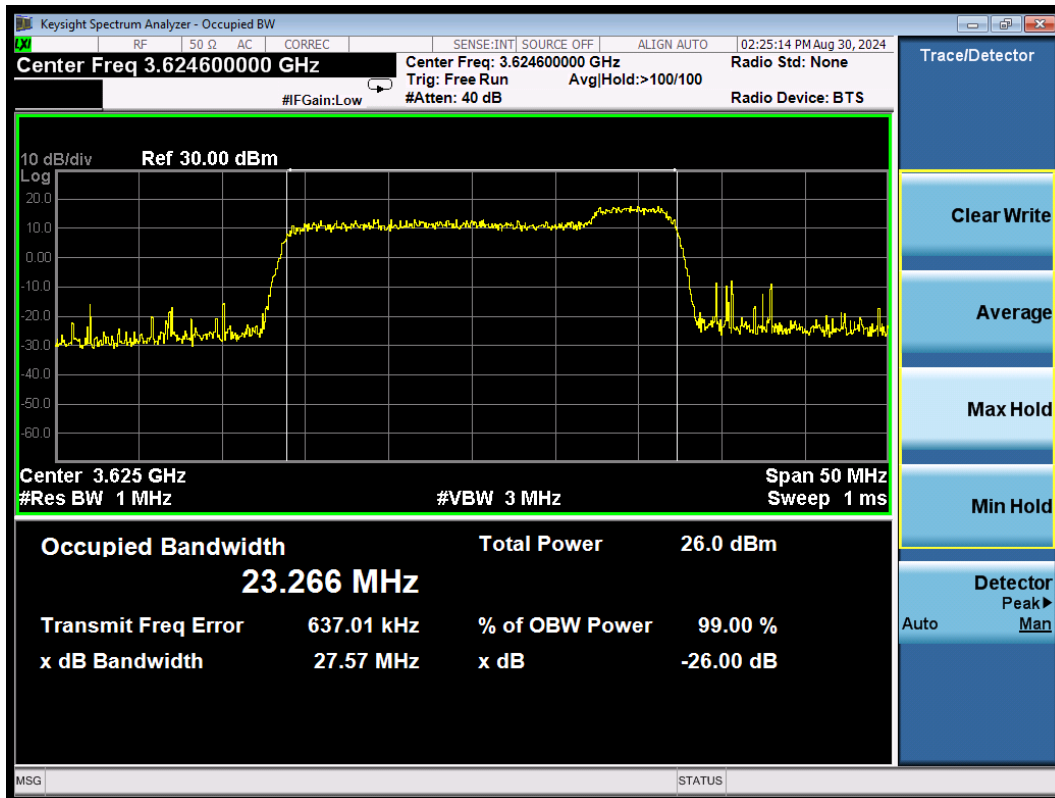
CA_48C 16QAM\20MHz+5MHz Middle
