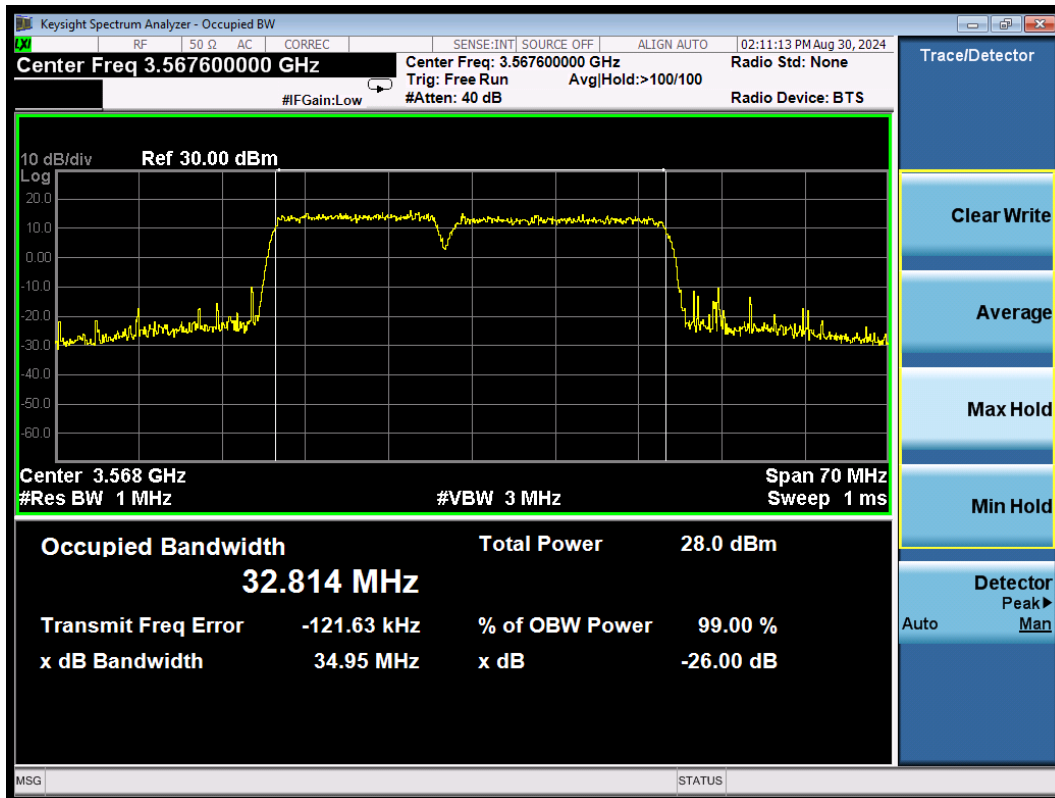
CA_48C QPSK\15MHz+20MHz Low
