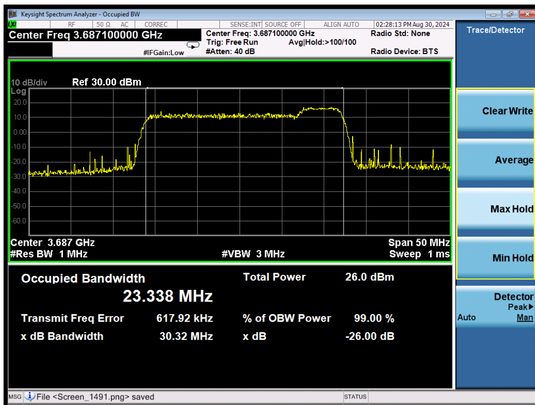
CA_48C QPSK\20MHz+5MHz High
