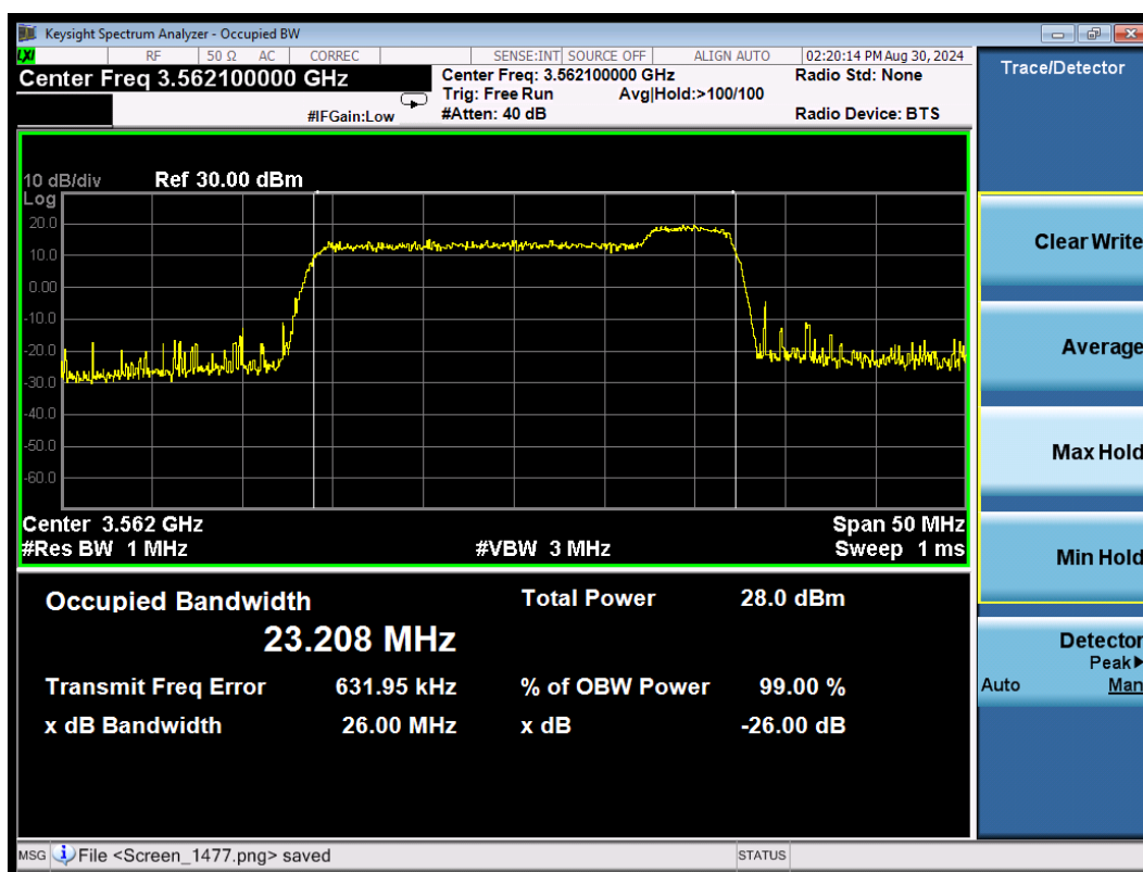
CA_48C 64QAM\20MHz+5MHz Low
