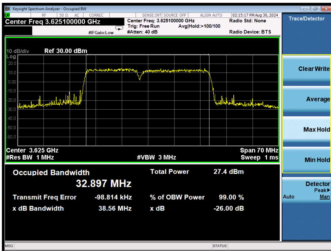
CA_48C QPSK\15MHz+20MHz Middle
