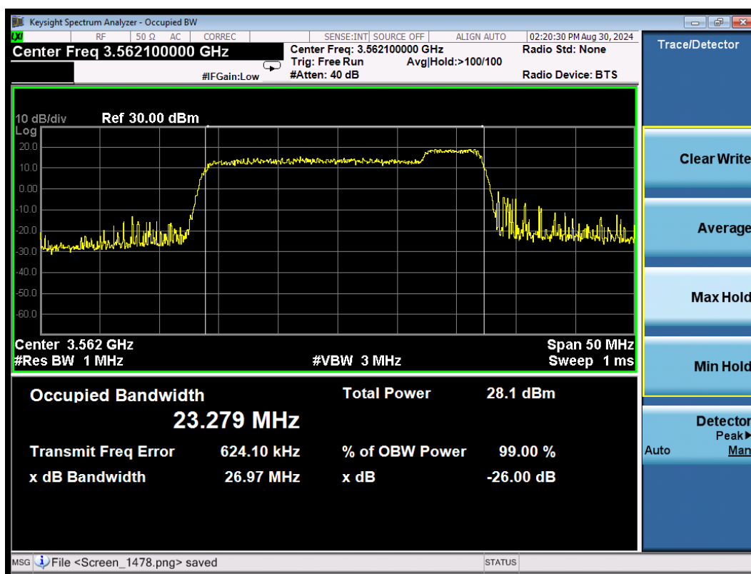
CA_48C 16QAM\20MHz+5MHz Low
