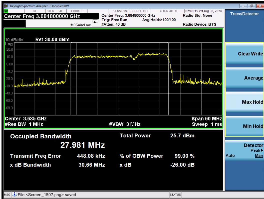
CA_48C 64QAM\20MHz+10MHz High
