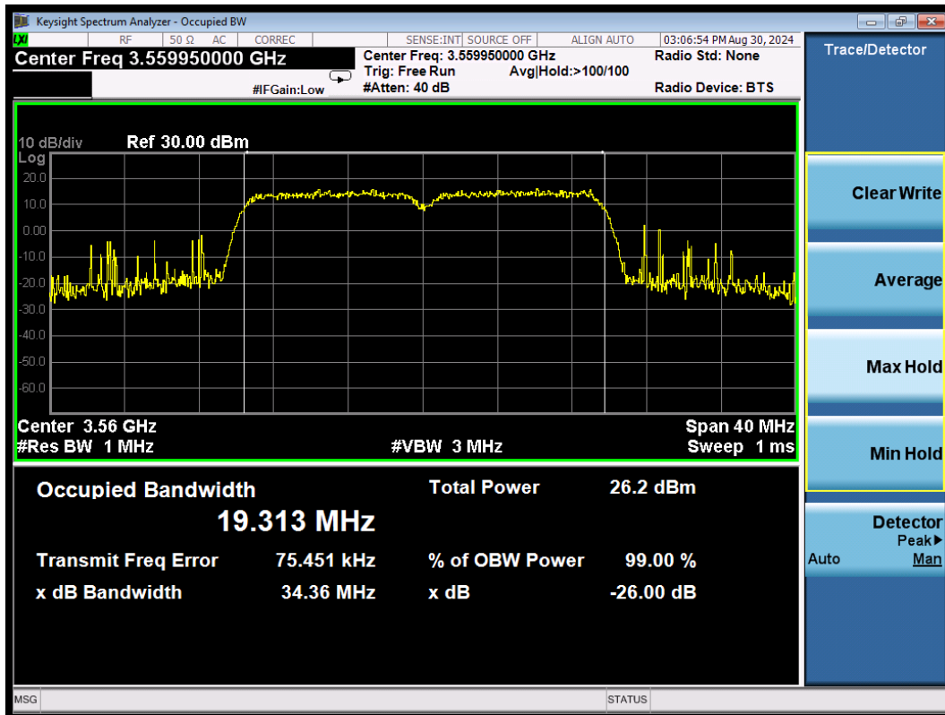
CA_48B 256QAM\10MHz+10MHz Low
