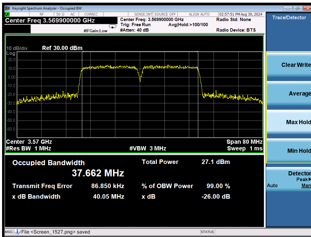
CA_48C 16QAM\20MHz+20MHz Low
