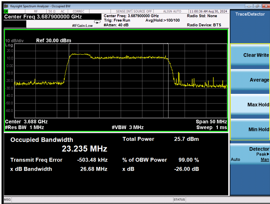
CA_48C QPSK\5MHz+20MHz High
