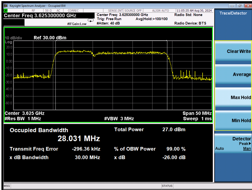
CA_48C QPSK\10MHz+20MHz Middle
