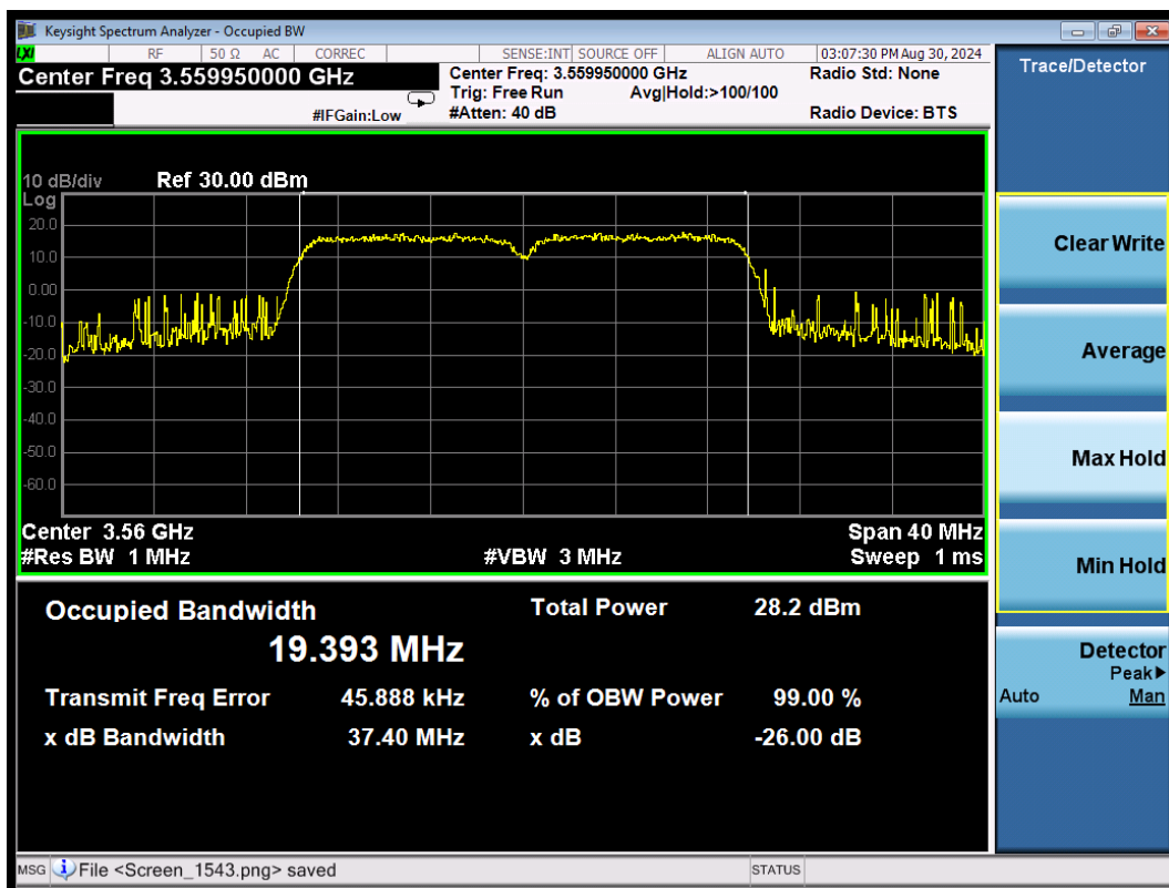
CA_48B 64QAM\10MHz+10MHz Low
