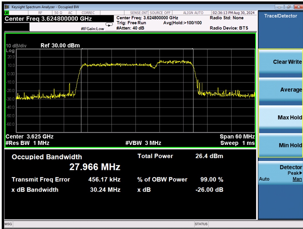
CA_48C 64QAM\20MHz+10MHz Middle
