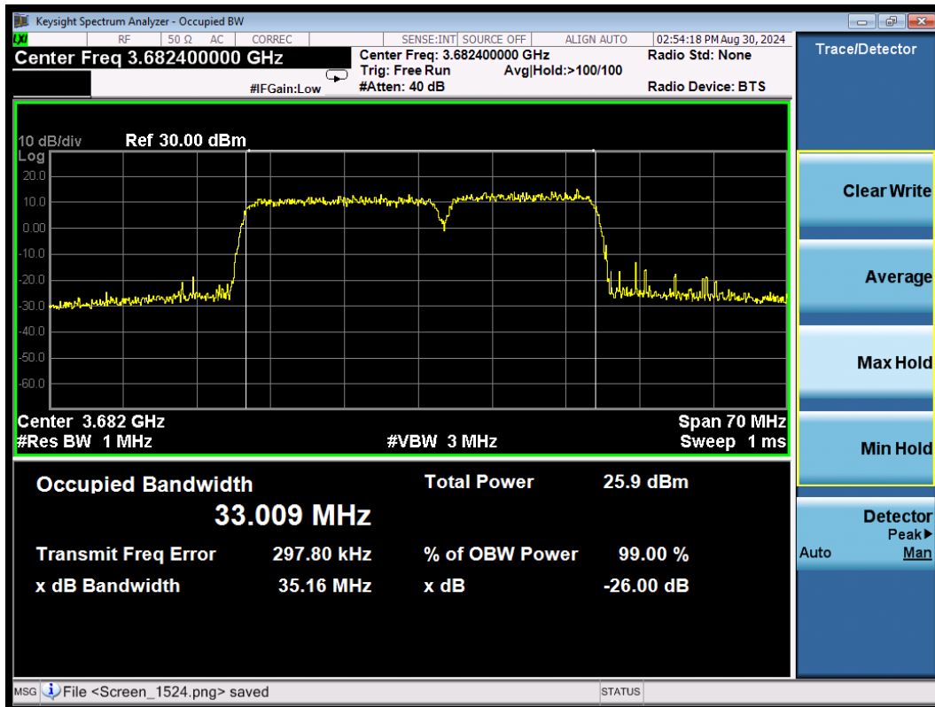
CA_48C 16QAM\20MHz+15MHz High
