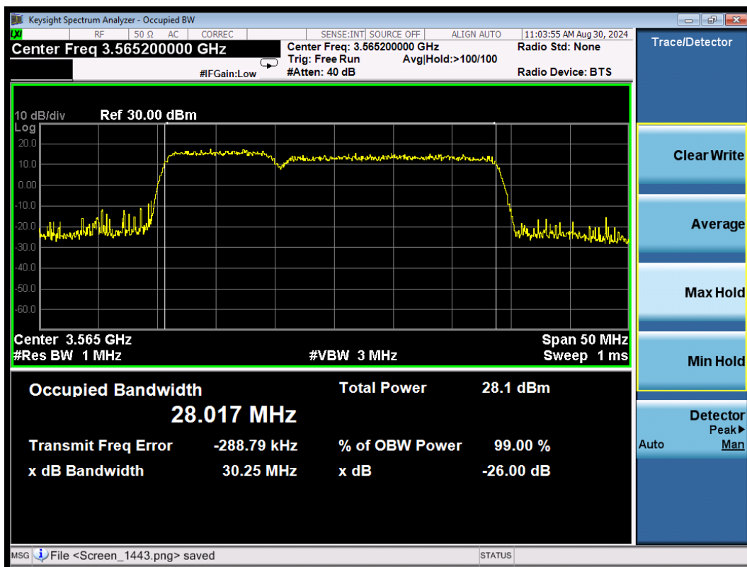
CA_48C 64QAM\10MHz+20MHz Low
