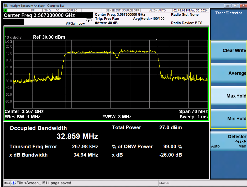
CA_48C 64QAM\20MHz+15MHz Low
