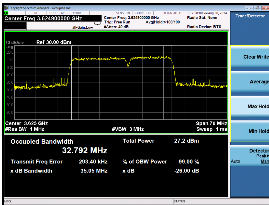
CA_48C QPSK\20MHz+15MHz Middle
