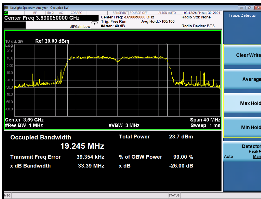
CA_48B 256QAM\10MHz+10MHz High
