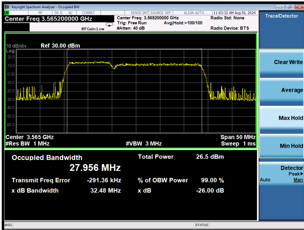
CA_48C 256QAM\10MHz+20MHz Low
