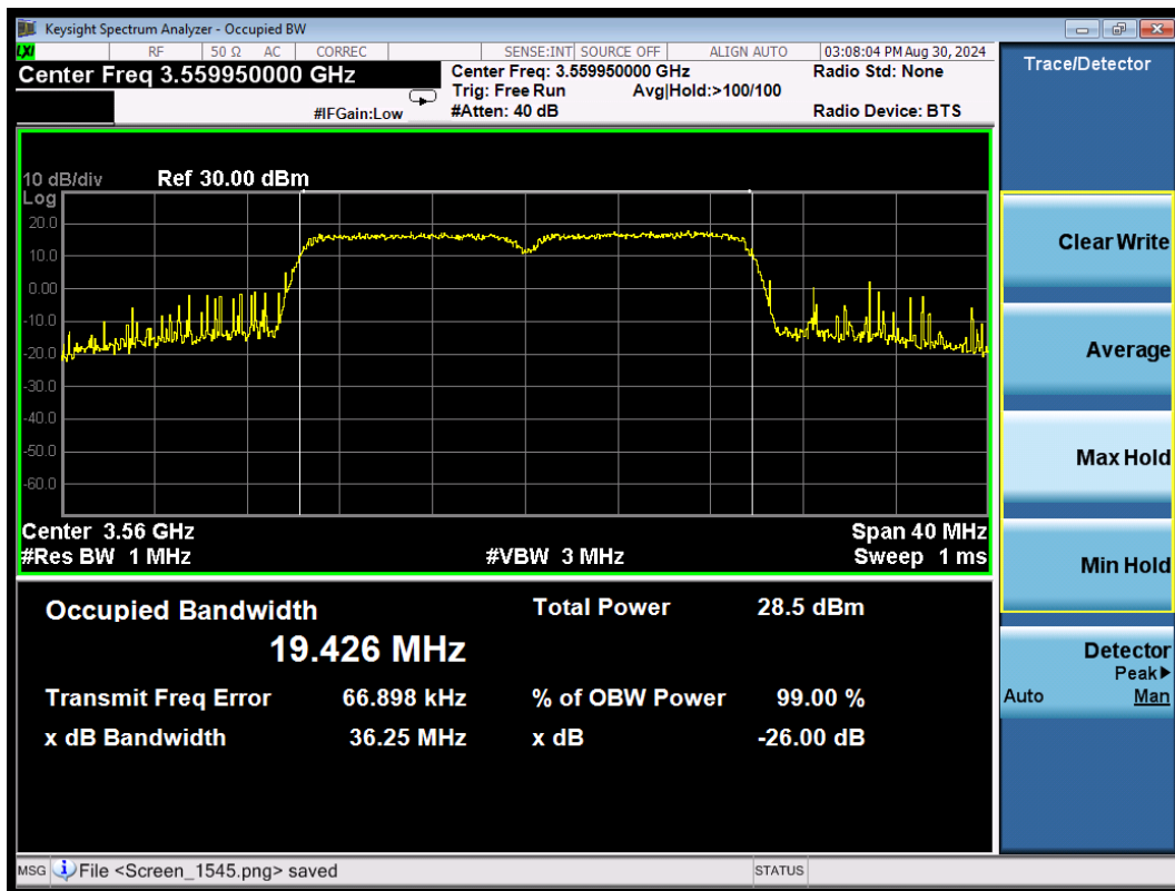
CA_48B QPSK\10MHz+10MHz Low
