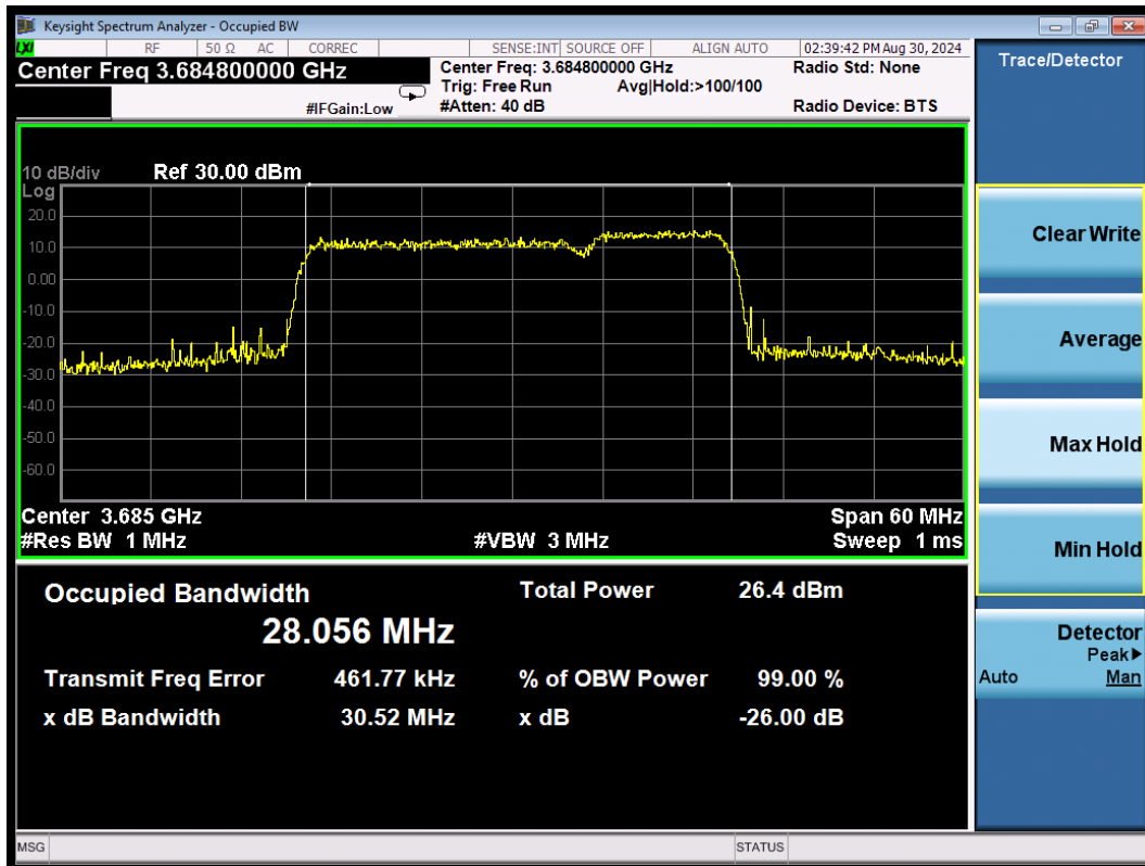
CA_48C QPSK\20MHz+10MHz High
