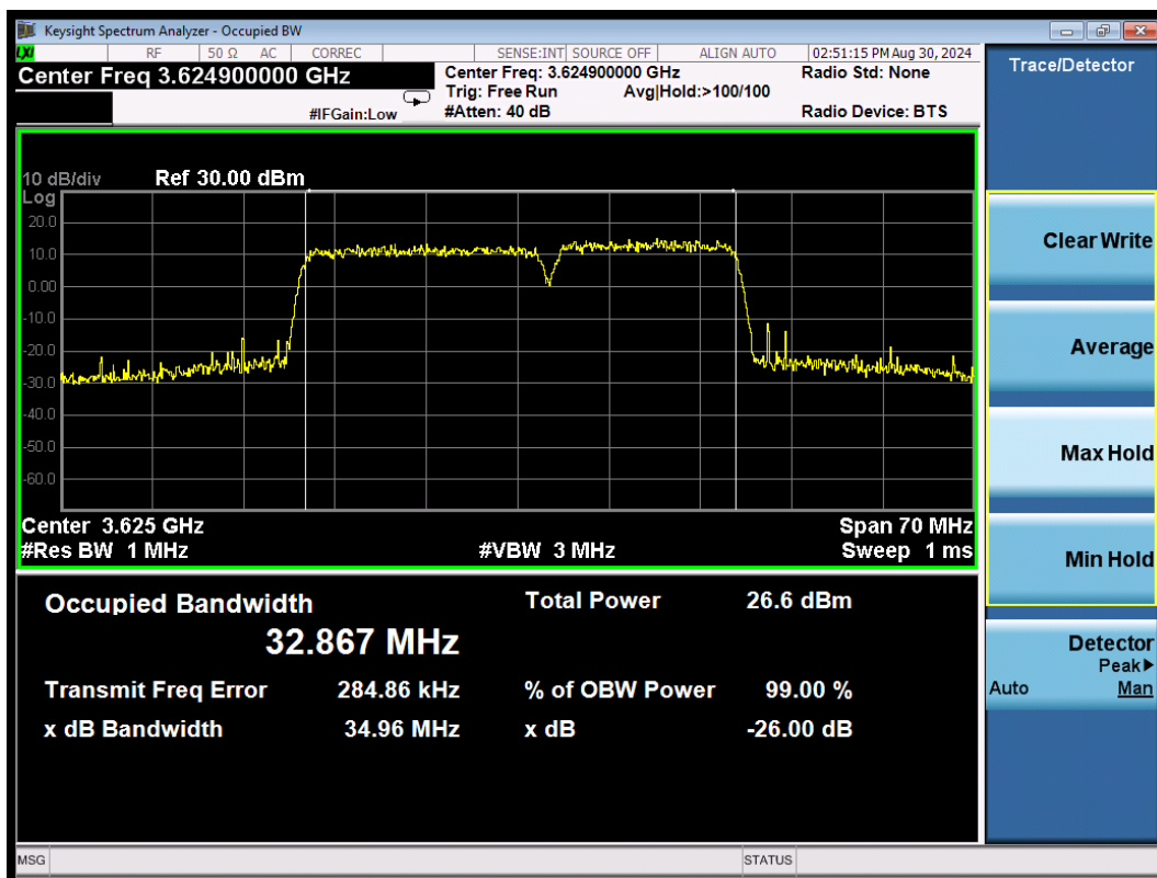
CA_48C 64QAM\20MHz+15MHz Middle
