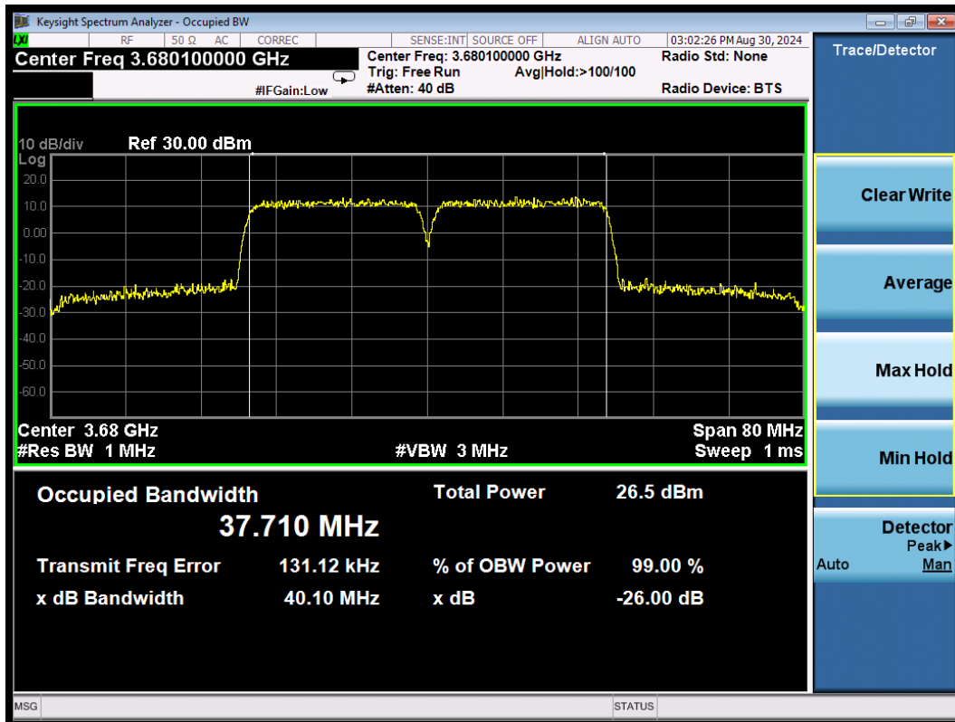
CA_48C QPSK\20MHz+20MHz High
