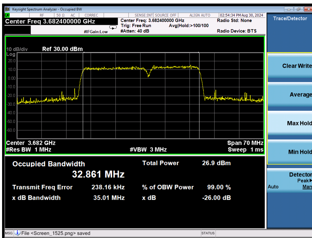
CA_48C QPSK\20MHz+15MHz High
