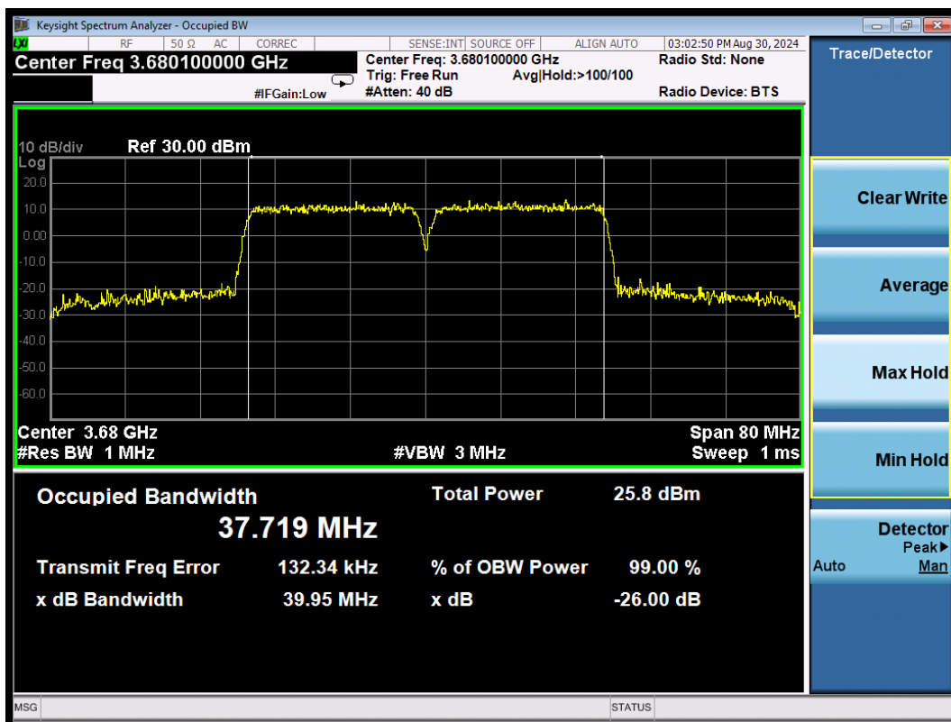
CA_48C 16QAM\20MHz+20MHz High
