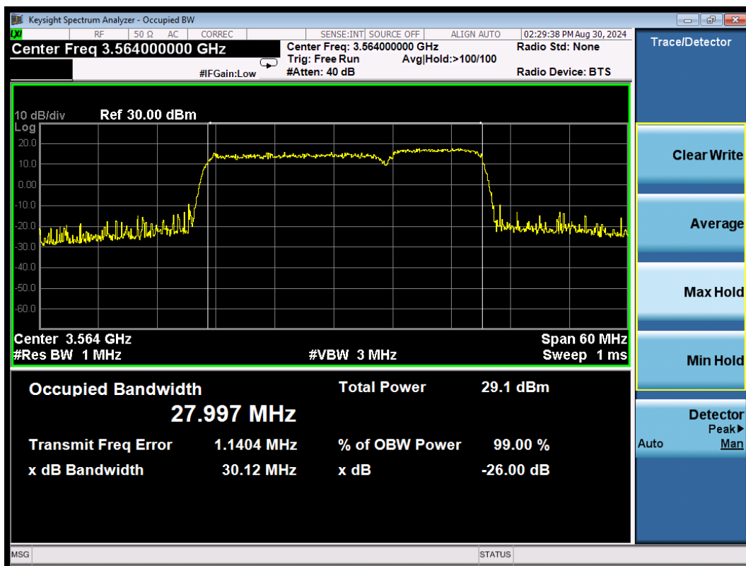
CA_48C QPSK\20MHz+10MHz Low
