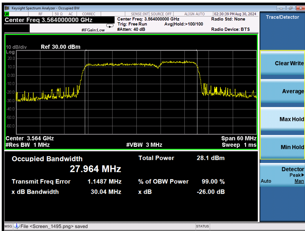
CA_48C 64QAM\20MHz+10MHz Low
