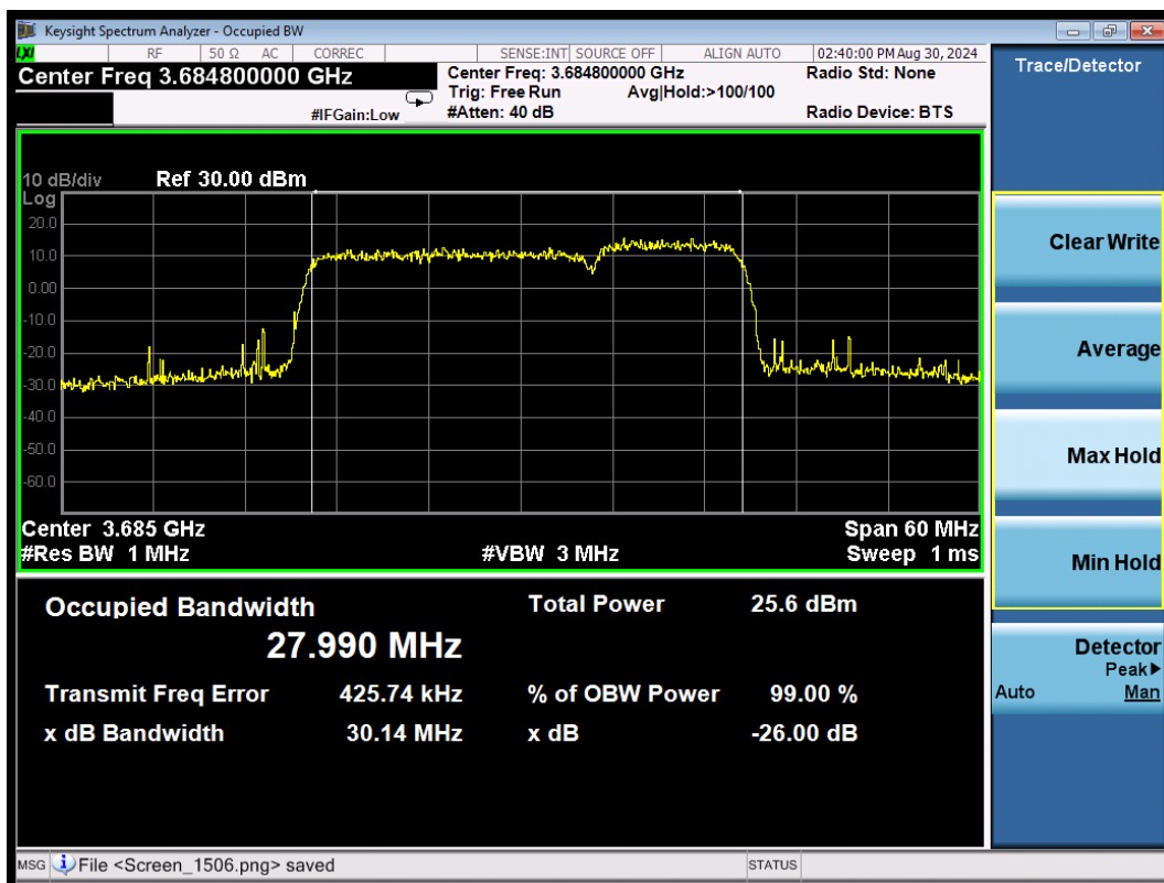
CA_48C 16QAM\20MHz+10MHz High
