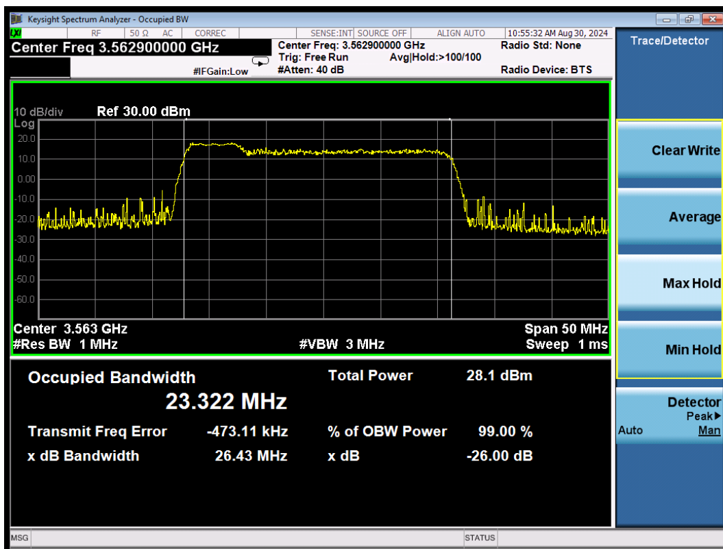
CA_48C QPSK\5MHz+20MHz Low
