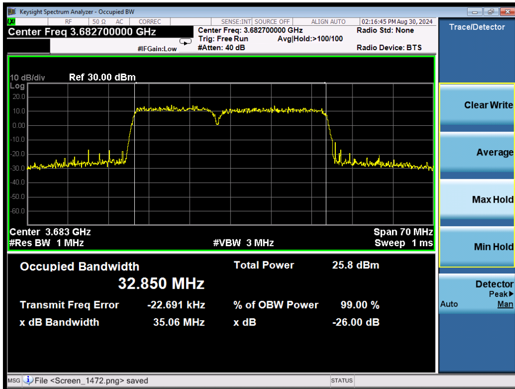
CA_48C 16QAM\15MHz+20MHz High
