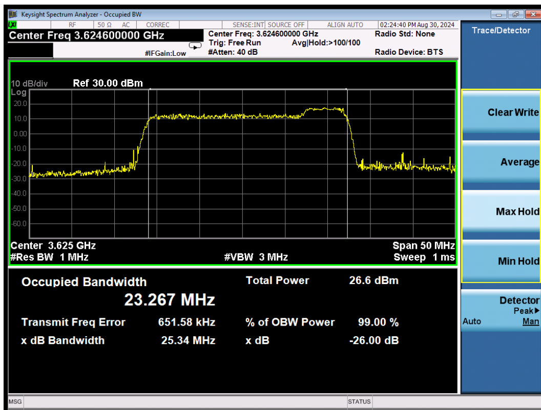
CA_48C QPSK\20MHz+5MHz Middle
