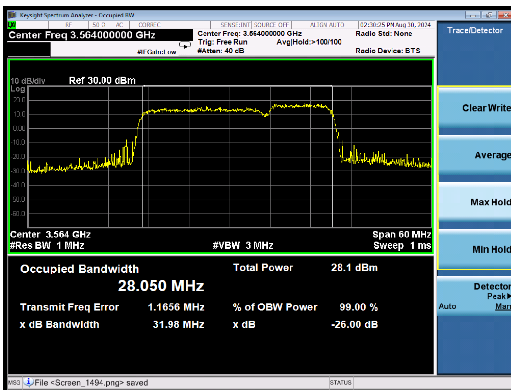
CA_48C 16QAM\20MHz+10MHz Low
