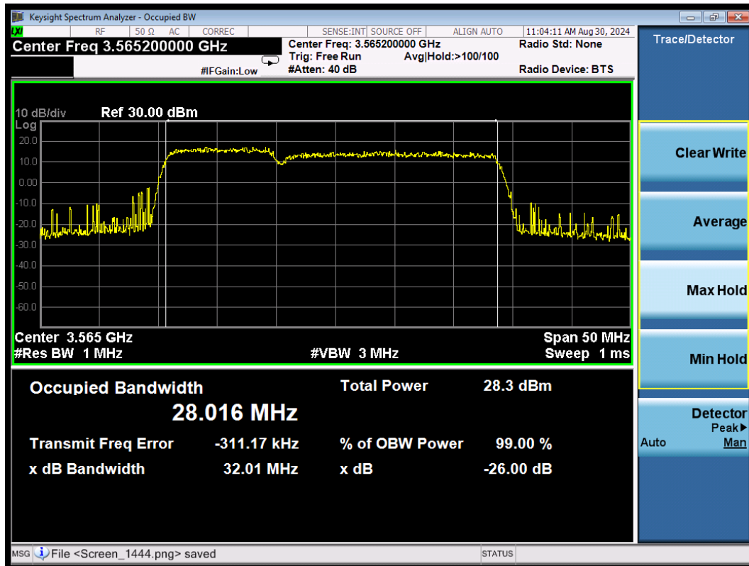
CA_48C 16QAM\10MHz+20MHz Low
