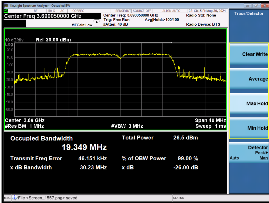
CA_48B QPSK\10MHz+10MHz High
