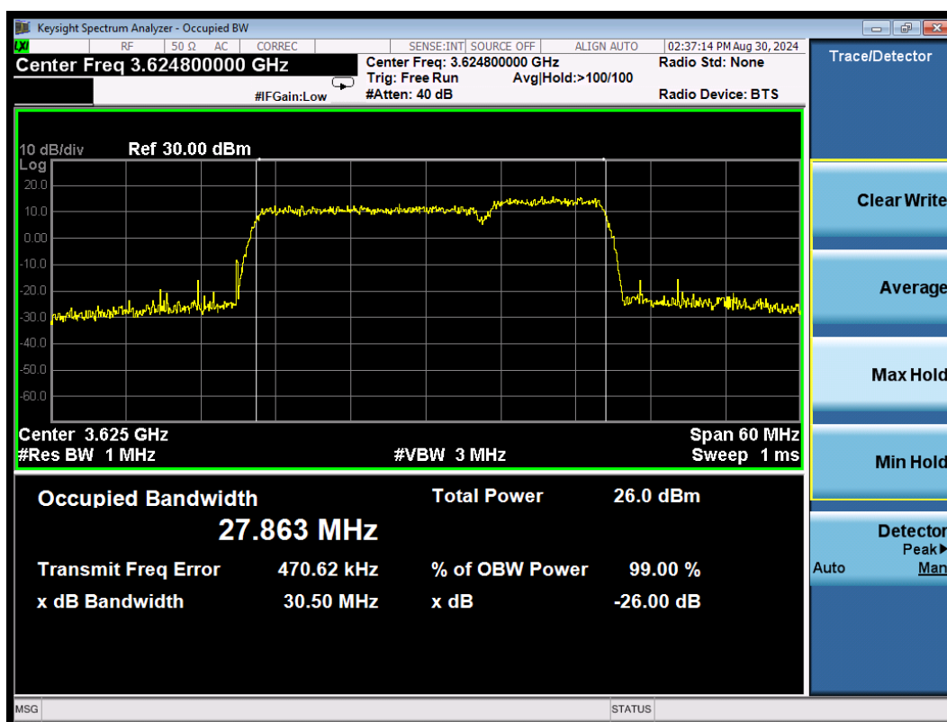
CA_48C 16QAM\20MHz+10MHz Middle
