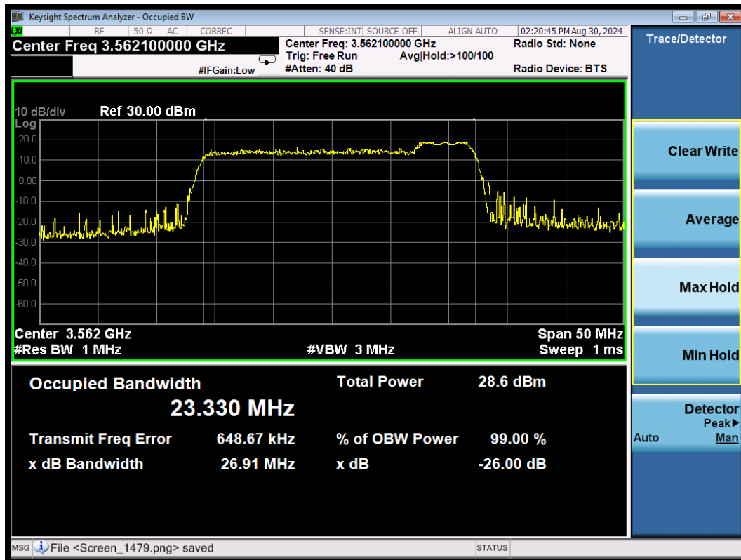
CA_48C QPSK\20MHz+5MHz Low
