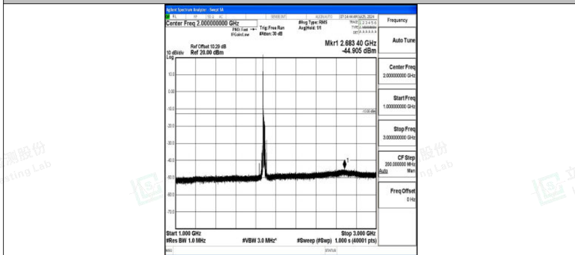
Band2-20MHz-QPSK-18900-1RB#0-1000~3000-PASS
