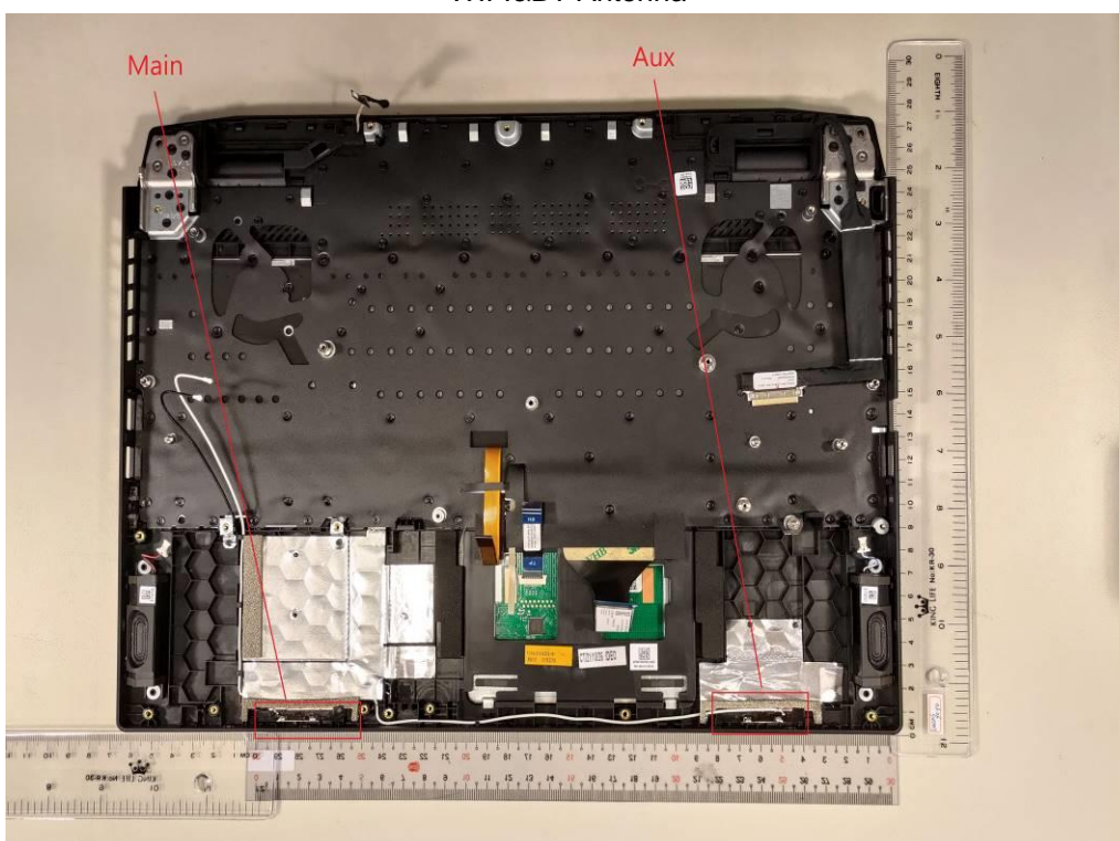
WIFI&BT Antenna
