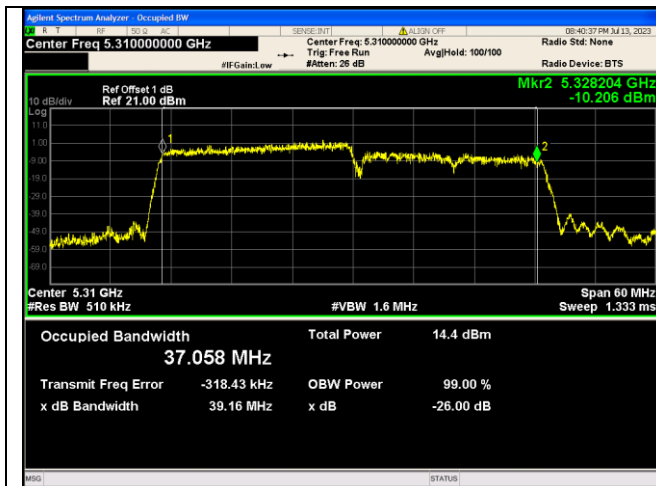
IEEE 802.11ax_Channel 62_40MHz_Antenna 0_RU&amp;Index 242RU61
