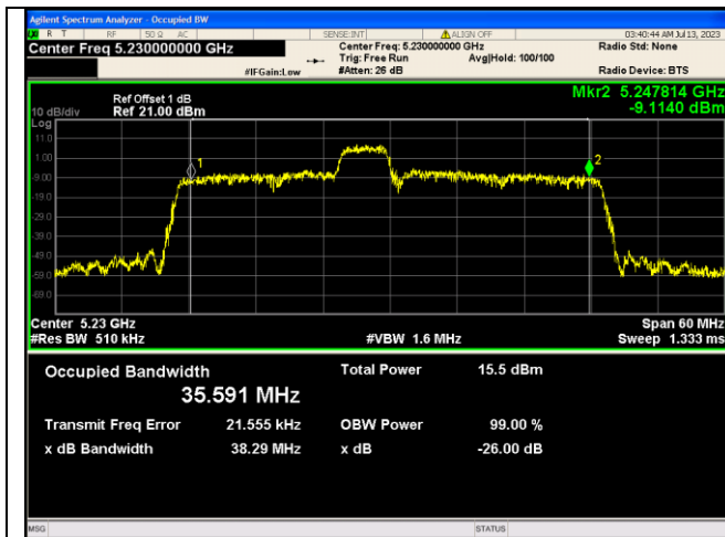
IEEE 802.11ax_Channel 46_40MHz_Antenna 0_RU&amp;Index 52RU40
