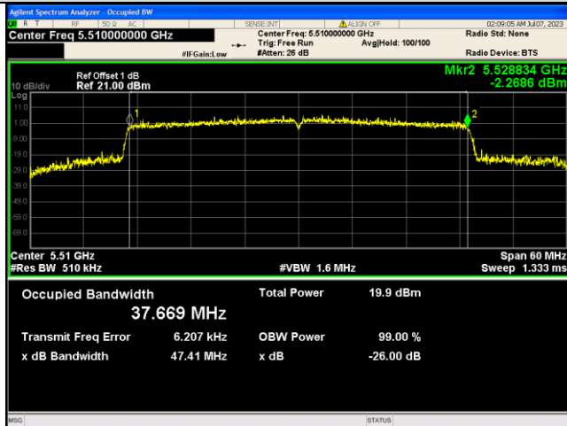
IEEE 802.11ax_Channel 102_40MHz_Antenna 0_RU&amp;Index 484RU65
