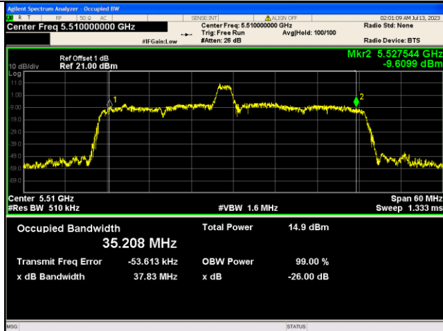
IEEE 802.11ax_Channel 102_40MHz_Antenna 0_RU&amp;Index 26RU8
