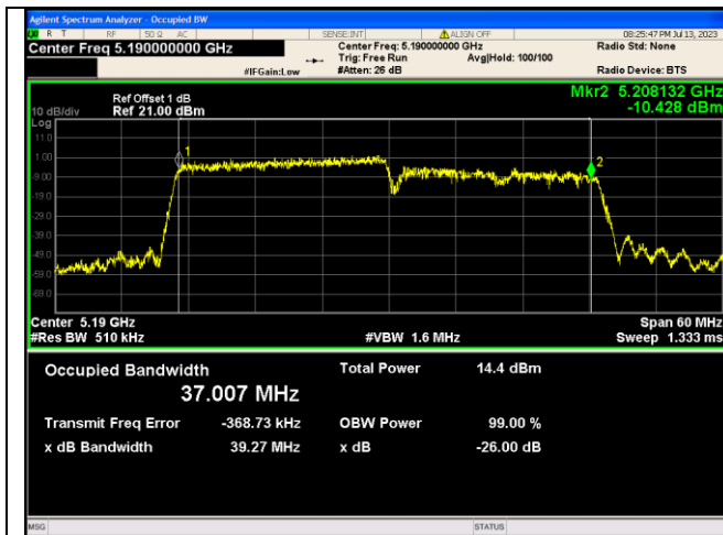
IEEE 802.11ax_Channel 38_40MHz_Antenna 0_RU&amp;Index 242RU61
