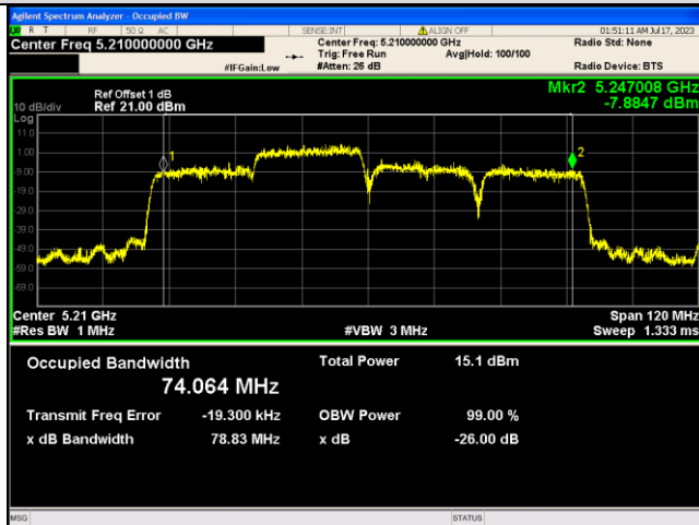
IEEE 802.11ax_Channel 42_80MHz_Antenna 0_RU&amp;Index 242RU62
