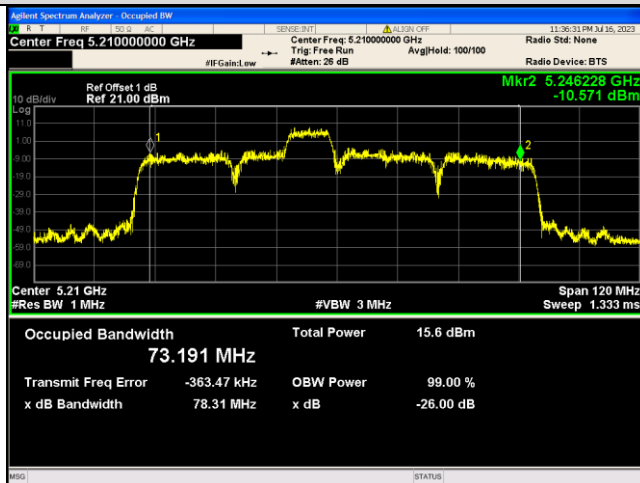
IEEE 802.11ax_Channel 42_80MHz_Antenna 0_RU&amp;Index 106RU56
