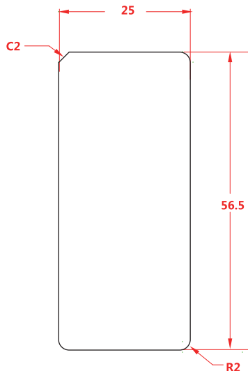
尺寸图
