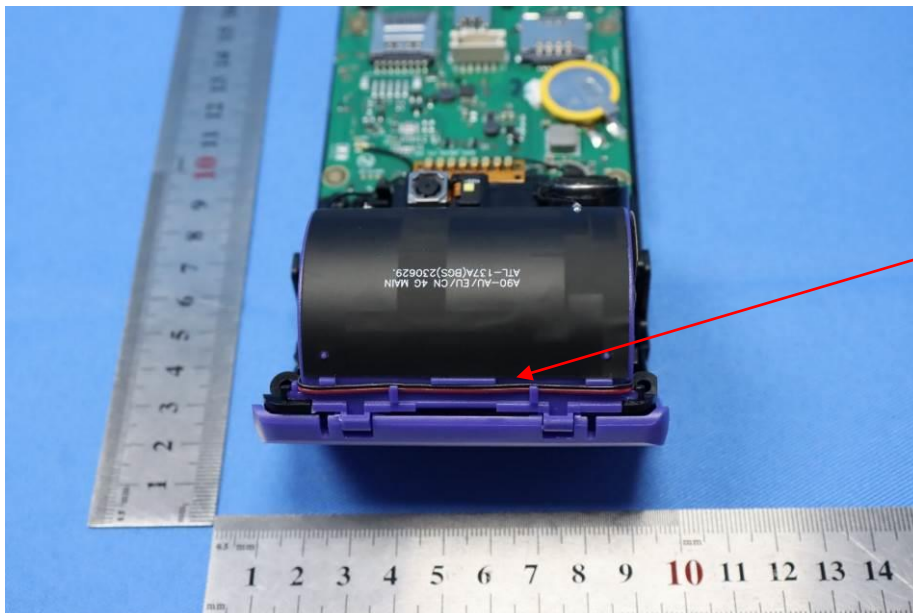
NFC antenna
