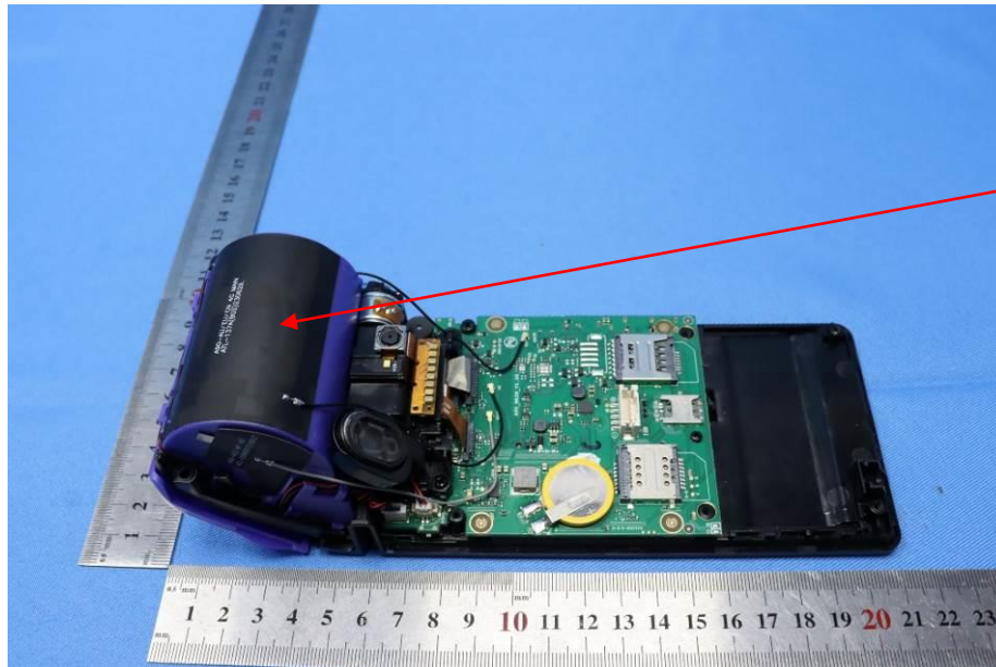
WWAN antenna
