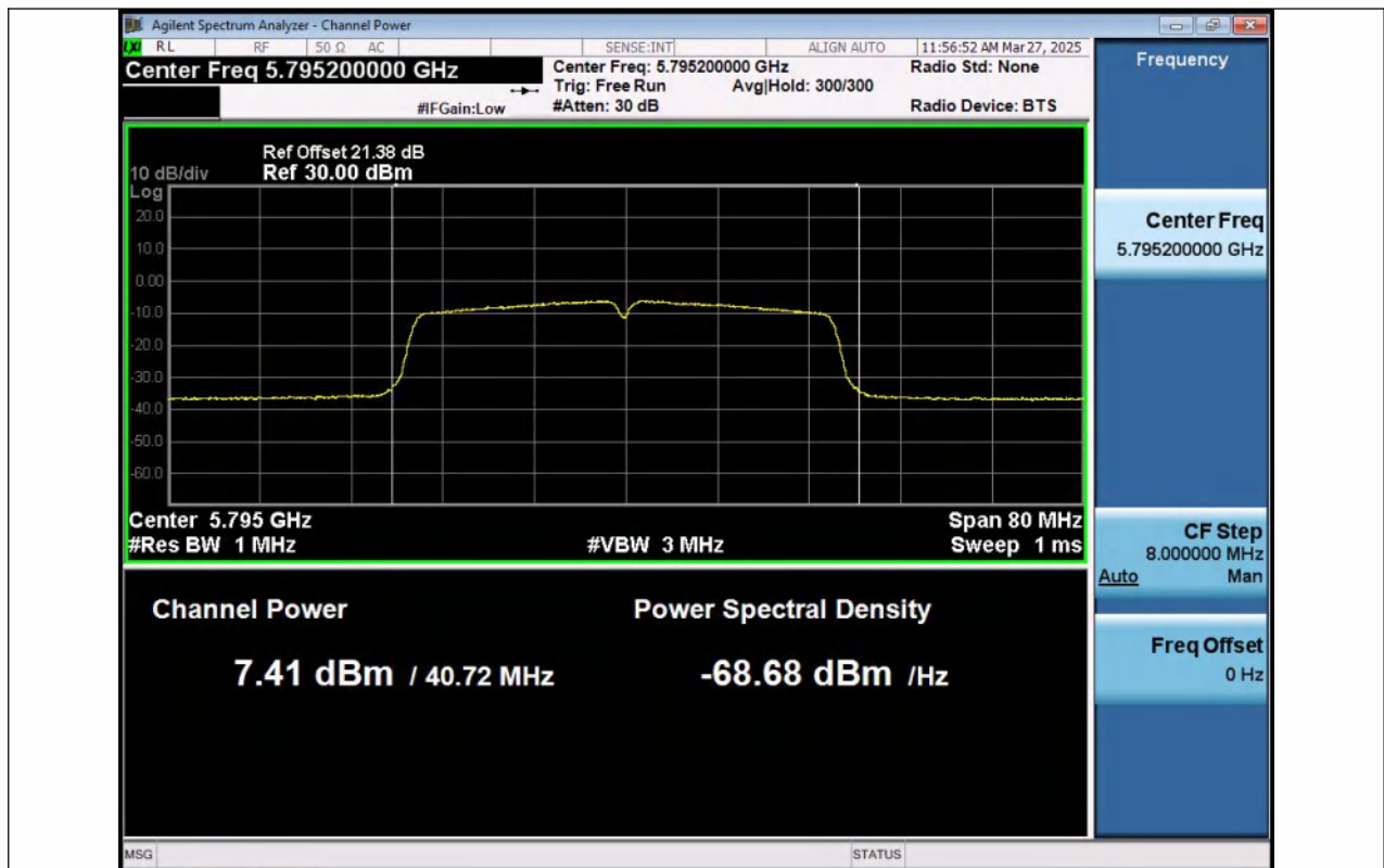
11N40MIMO-Ant1-5795-PASS
