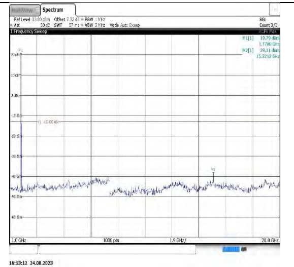
Band66-3MHz-QPSK-131987-1RB#0- Range2:1000~20000MHz
