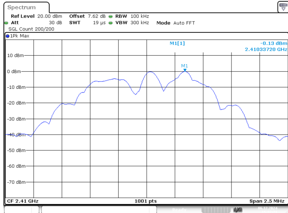
PSD NVNT GFSK 2410MHz Ant1
