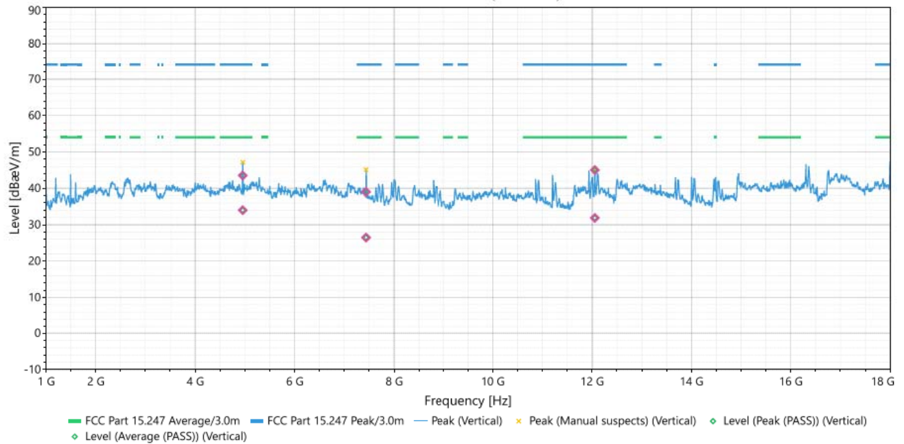
#1 - 1GHz-18GHz (Vertical)
