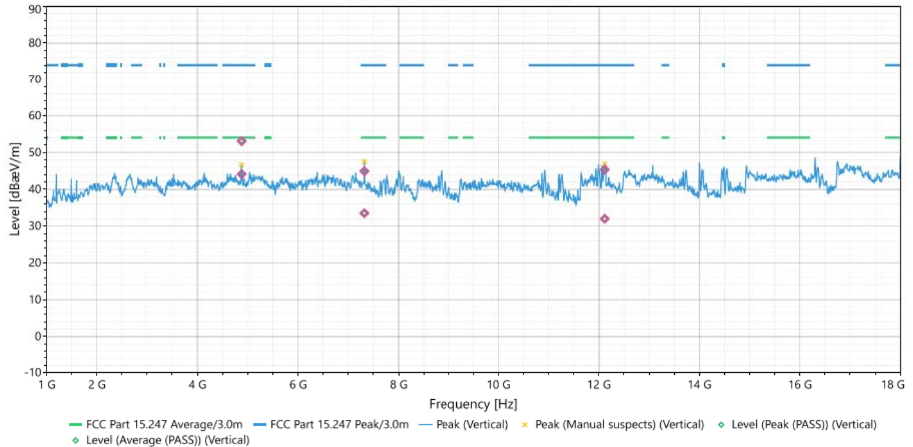
#1 - 1GHz-18GHz (Vertical)
