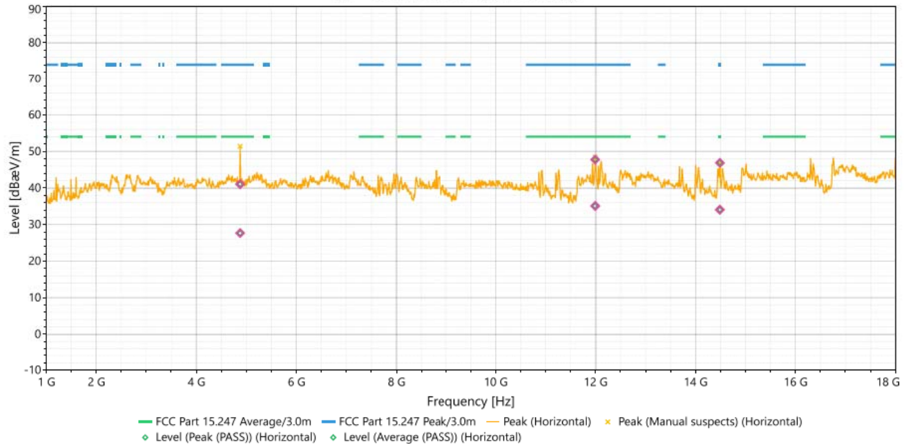
#2 - 1GHz-18GHz (Horizontal)
