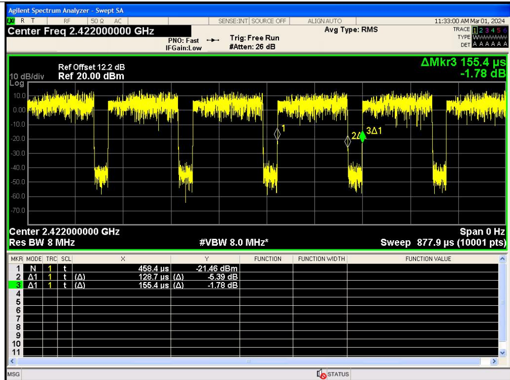
IEEE 802.11n_40MHz_Channel 3
