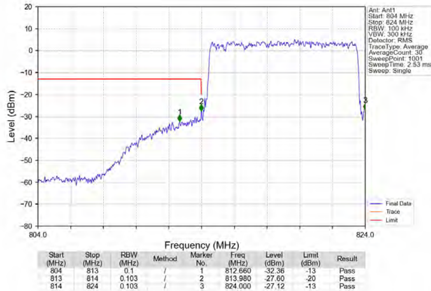
Band26a_10MHz_QPSK_LCH_819MHz_RB_50_0_NTNV
