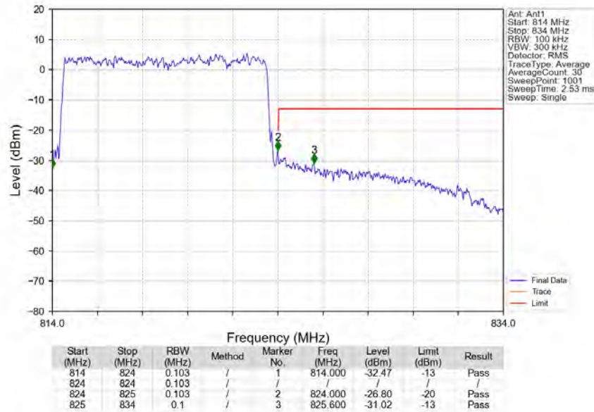
Band26a_10MHz_QPSK_HCH_819MHz_RB_1_0_NTNV
