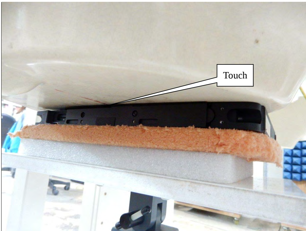
EUT Back-Main
