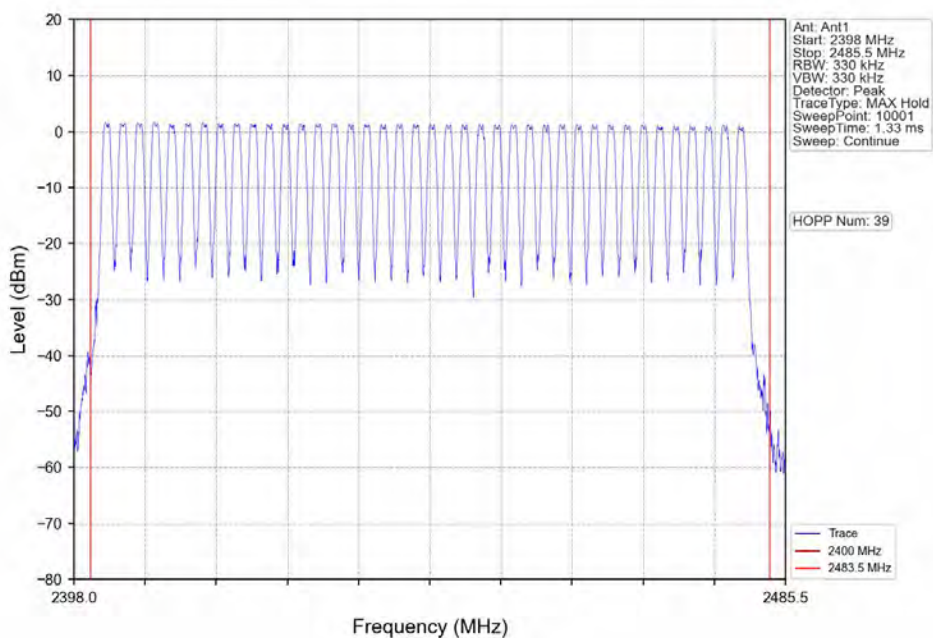
PI/4-QDPSK_HOPP_Ant1_NTNV
