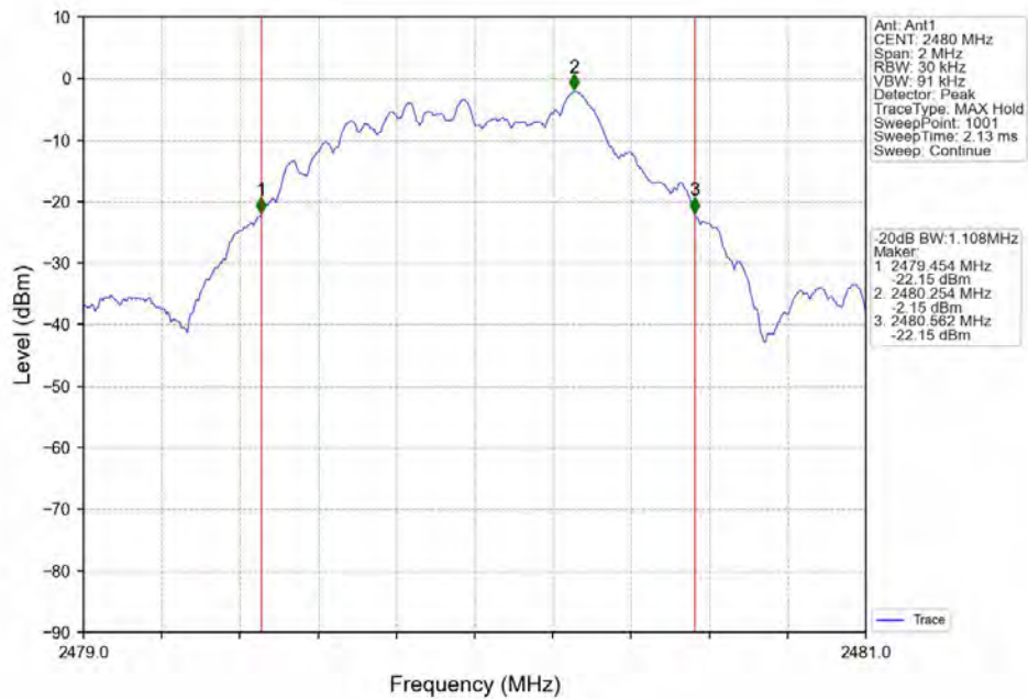
PI/4-QDPSK_HCH_2480MHz_Ant1_NTNV
