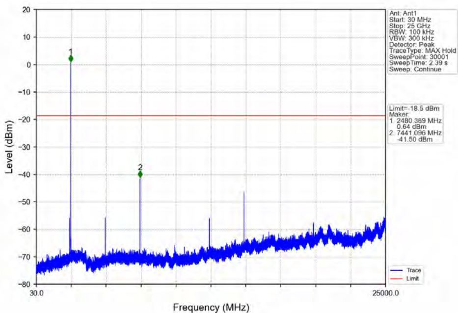
PI/4-QDPSK_HCH_2480MHz_Ant1_NTNV
