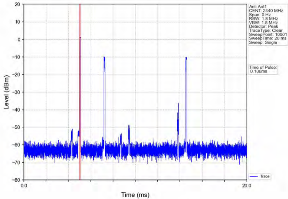
PI/4-QDPSK_HOPP_Ant1_NTNV
