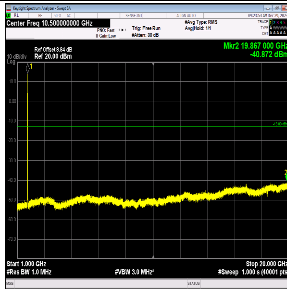
Band4-1413-4-1000~20000MHz-PASS
