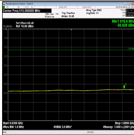
Band4-1513-4-30~1000MHz-PASS
