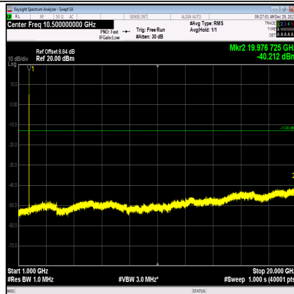
Band4-1413-5-1000~20000MHz-PASS
