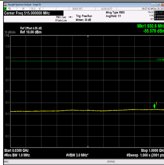
Band4-1513-5-30~1000MHz-PASS
