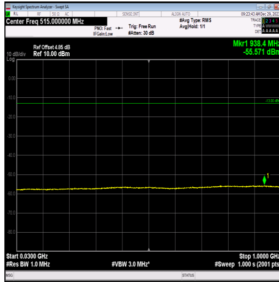
Band4-1413-4-30~1000MHz-PASS
