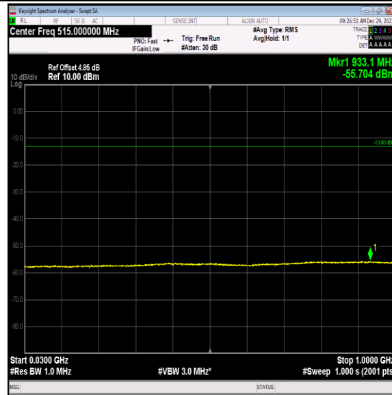
Band4-1413-5-30~1000MHz-PASS
