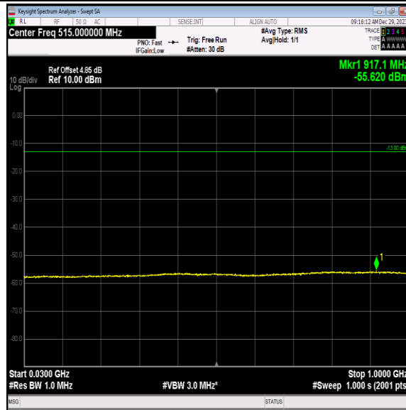
Band4-1413-2-30~1000MHz-PASS
