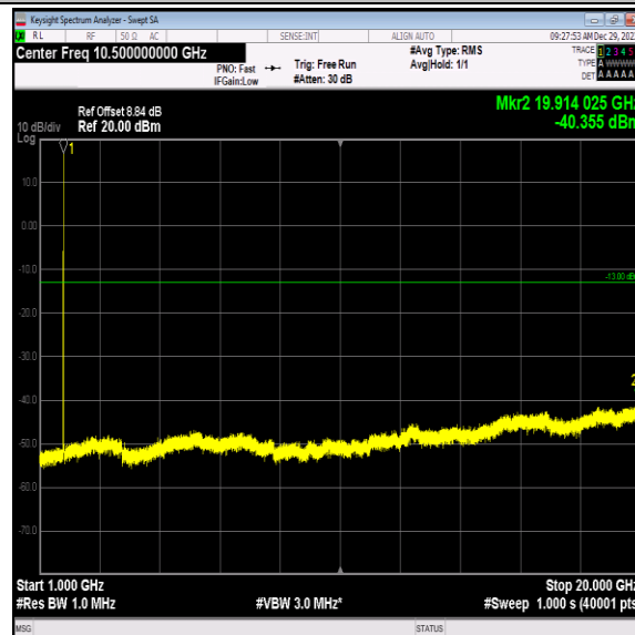
Band4-1513-5-1000~20000MHz-PASS
