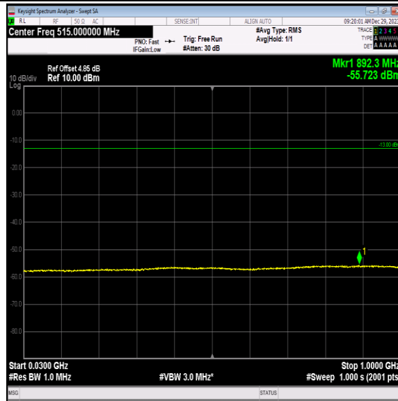
Band4-1413-3-30~1000MHz-PASS
