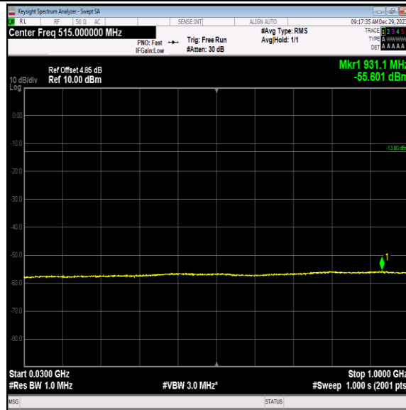
Band4-1513-2-30~1000MHz-PASS
