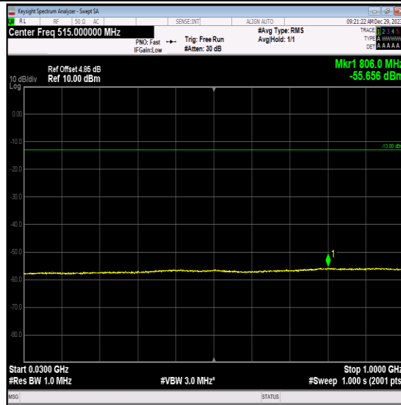
Band4-1513-3-30~1000MHz-PASS
