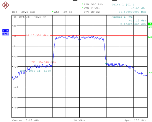
802.11ac40_5270MHz_Chain 1
