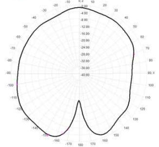
2440.0MHz Total(E1-XZ), Max=-0.90dBi
