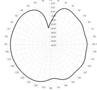
2400.0MHz Total(E2-YZ), Max=-3.04dBi
