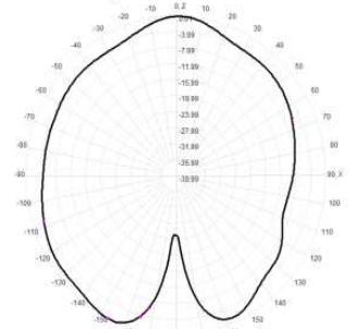
2480.0MHz Total(E1-XZ), Max=0.01dBi
