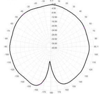
2440.0MHz Total(E2-YZ), Max=-2.05dBi
