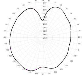
2400.0MHz Total(E1-XZ), Max=-0.97dBi
