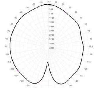
2480.0MHz Total(E2-YZ), Max=-0.23dBi
