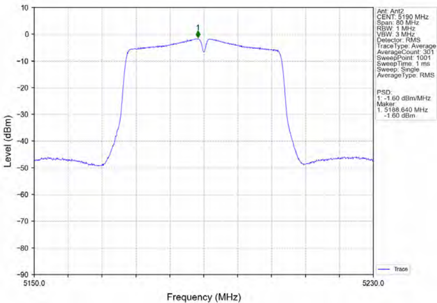
802.11n(HT40)_LCH_5190MHz_Ant2_NTNV
