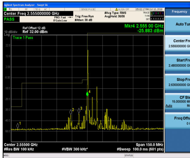
Band41_10MHz_QPSK_40290_1RB#0
