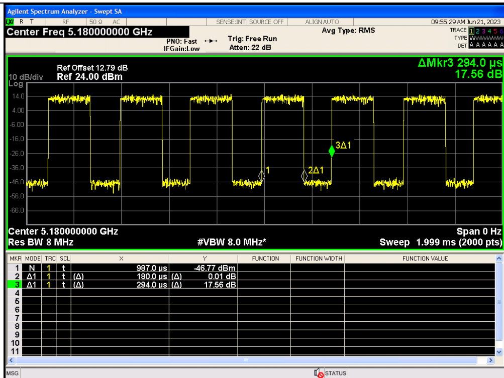
IEEE 802.11a_20MHz_Channel 36
