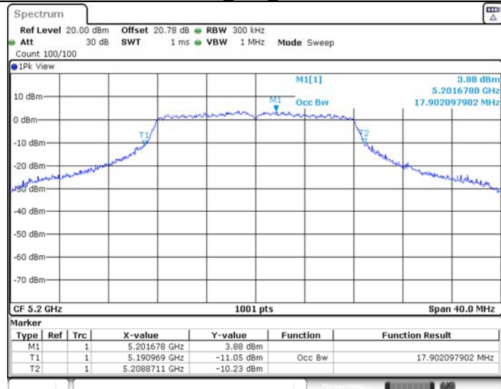
11A_Ant1_5200
