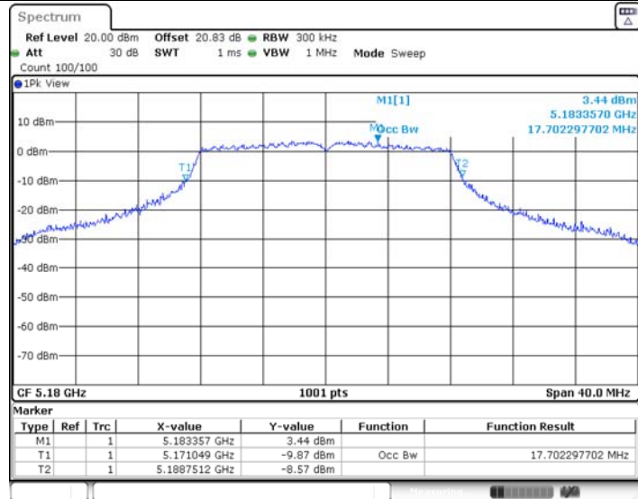
11A_Ant1_5180
