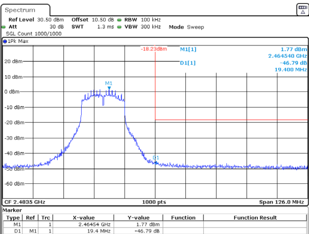
802.11n20_2462MHz_Chain 1
