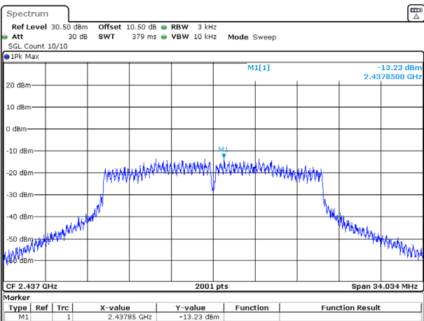
802.11n20_2437MHz_Chain 1
