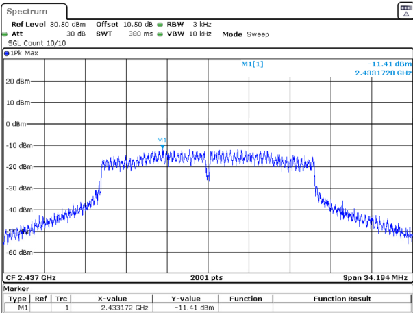
802.11n20_2437MHz_Chain 0
