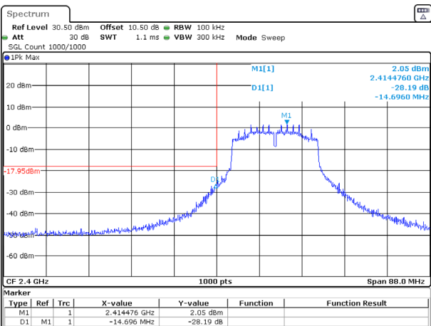
802.11n20_2412MHz_Chain 1
