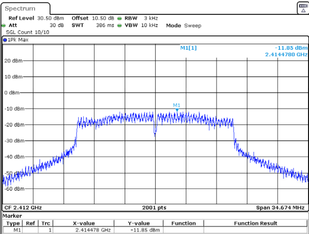
802.11n20_2412MHz_Chain 0
