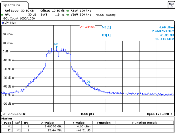
802.11n20_2462MHz_Chain 0
