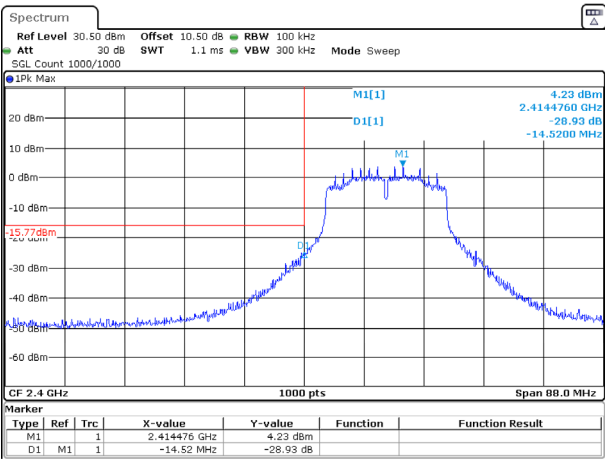
802.11n20_2412MHz_Chain 0
