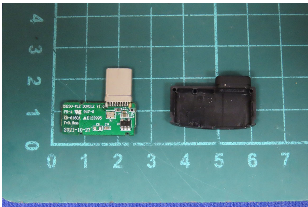
(9) EUT Photo
