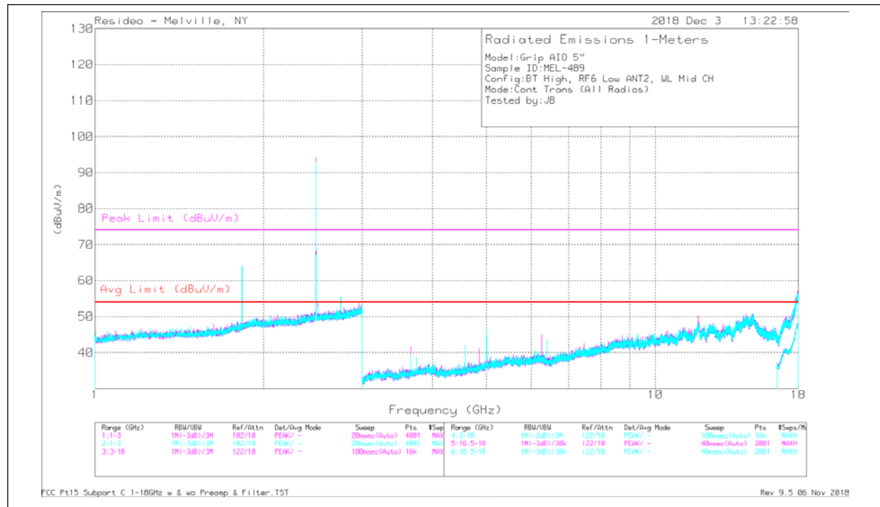
1-18GHz – Plot
