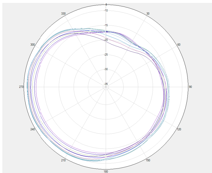
GSM850 / WCDMA B5 / LTE B5/B20 \Theta=90^\circ
