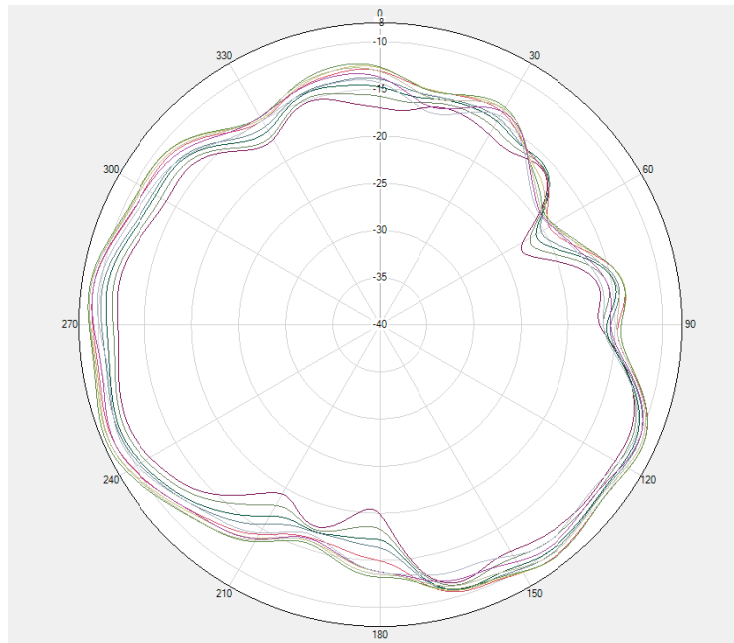
GSM850 / WCDMA B5 / LTE B5/B20 \Phi=90^\circ
