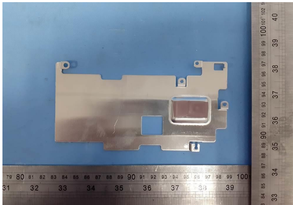
EUT Photo (4)
