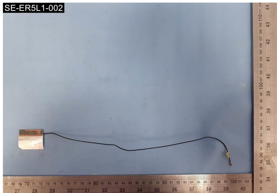
EUT Photo (30)
