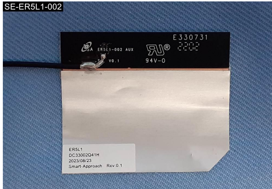
EUT Photo (30)
