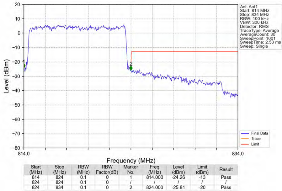
Band26a_10MHz_QPSK_MCH_819MHz_RB_50_0_NTNV
