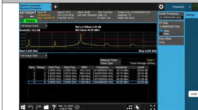
Band38-20MHz-QPSK-38150-1RB#99-PASS
