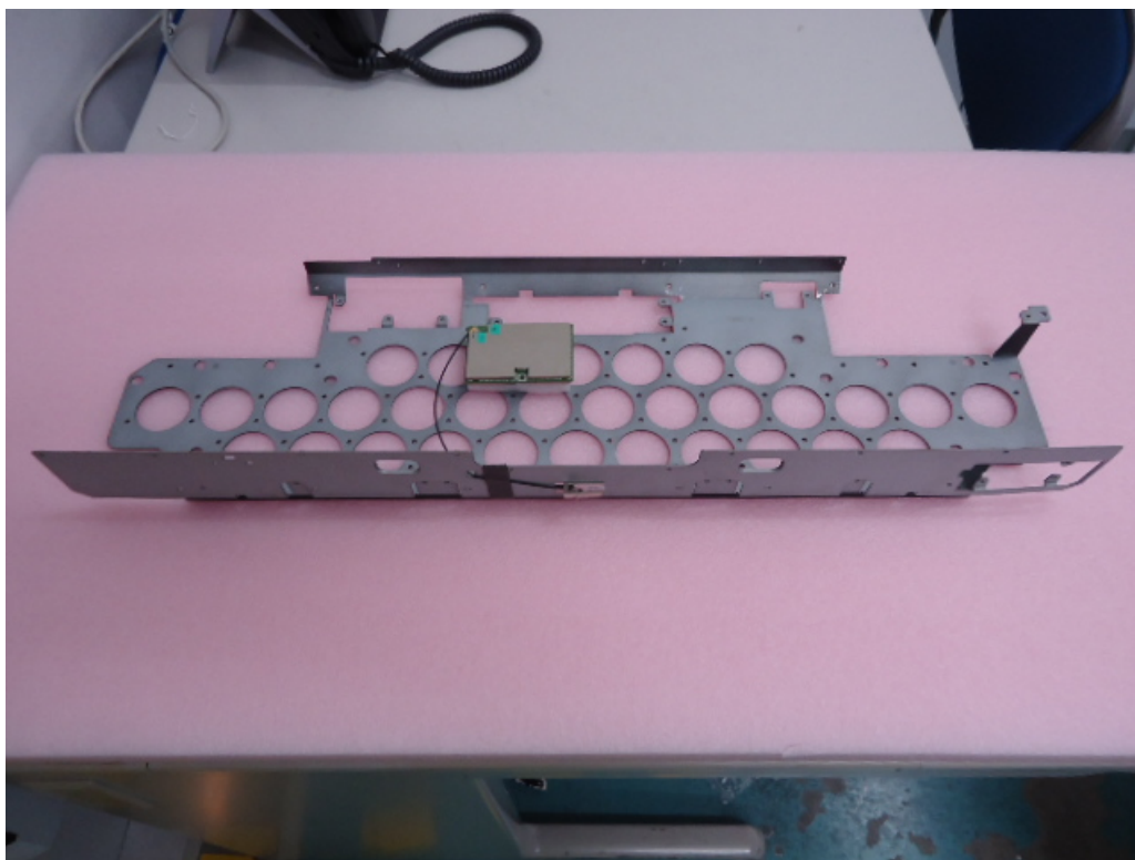
81EAY15.G09(PIFA) Whole
