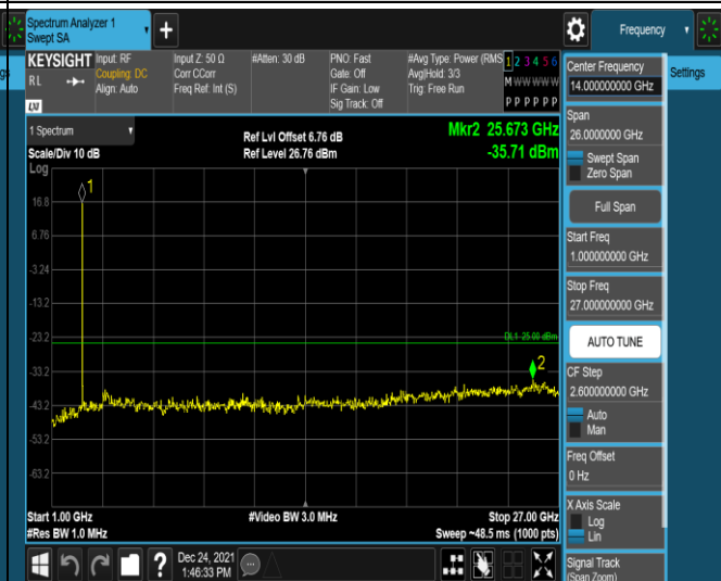
Band7-20MHz-QPSK-20850-1RB#0-Range2:1000~27 000MHz
