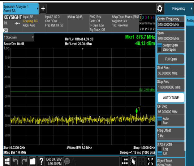
Band7-20MHz-QPSK-20850-1RB#0-Range1:30~1 000MHz
