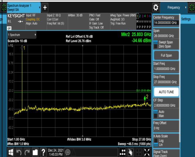
Band7-5MHz-16QAM-21425-1RB#0-Range2:1000~27 000MHz
