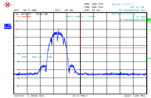
b_2462MHz_Chain 0 50.11dB
