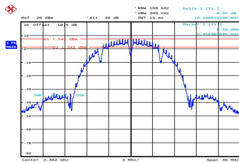
b_2462MHz_Chain 0 10.190MHz
