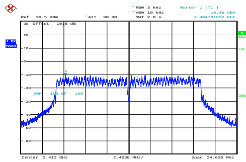
n20_2412MHz_Chain 0 -10.46dBm/3kHz
