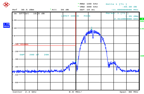
b_2412MHz_Chain 0 40.30dB
