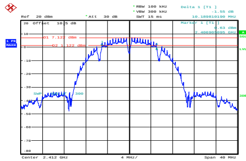
b_2412MHz_Chain 0 10.190MHz
