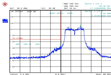
n20_2412MHz_Chain 0 30.36dB
