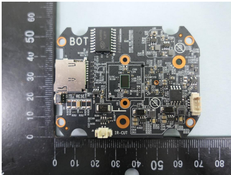
(15) EUT Photo
