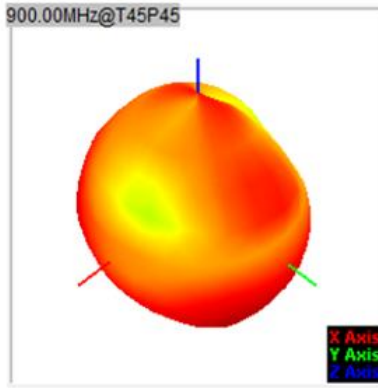
900.00MHz@T45P45
