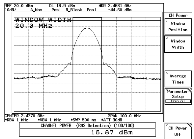
11Mbps-CH 06
