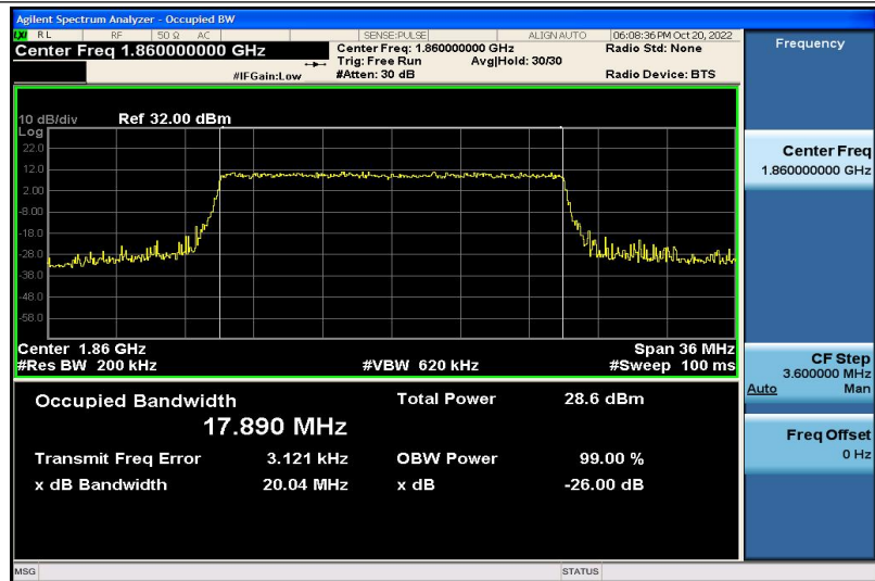
Band2-20MHz-QPSK-18700-100RB#0-17.890
