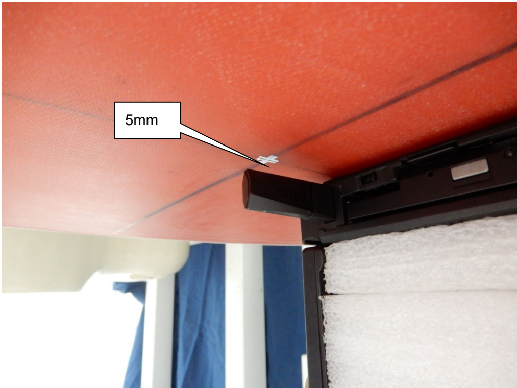
EUT Right-side(NB)
