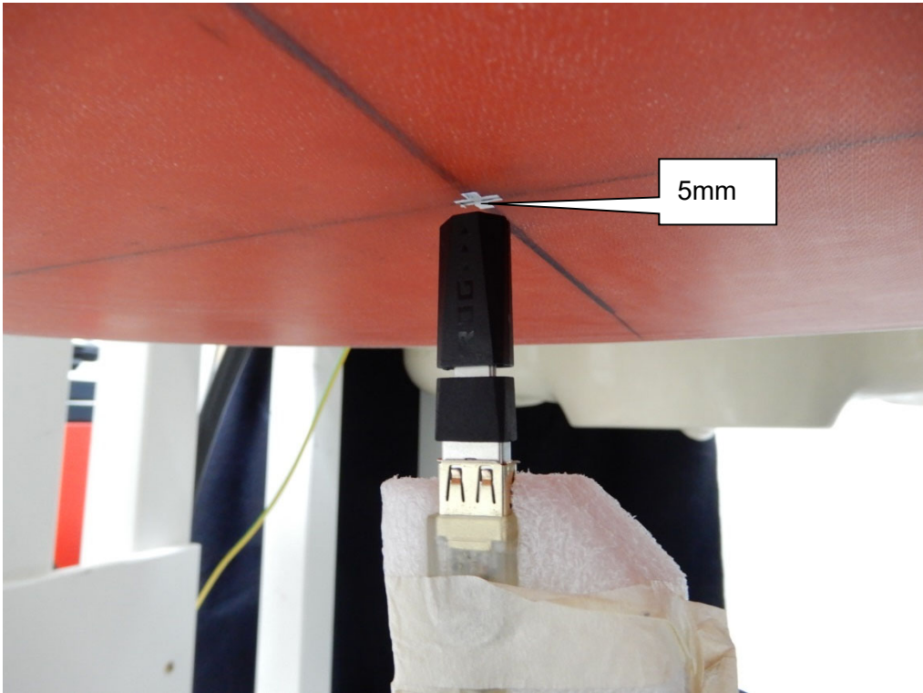
EUT Tip
