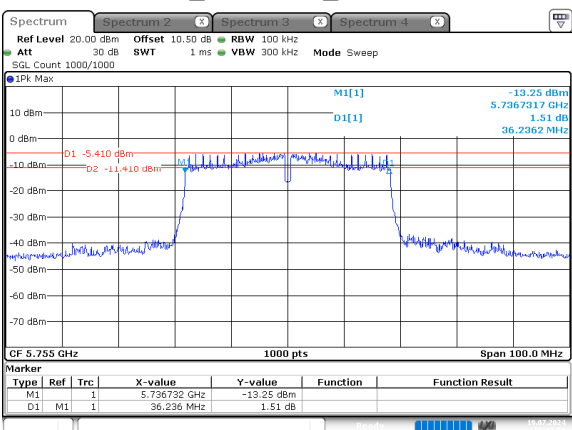
n40_5755MHz_Chain 0
