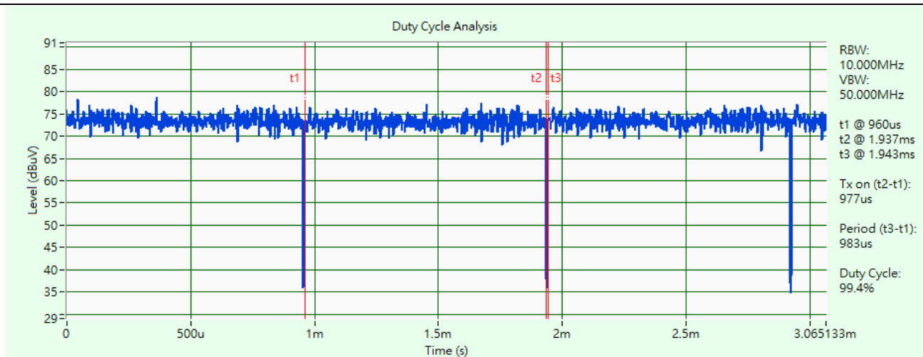
802.11ac (VHT20)
