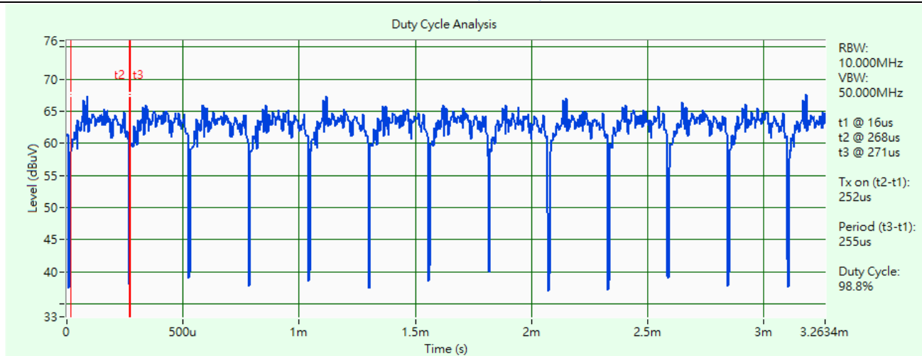
802.11ac (VHT80)
