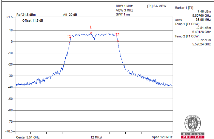
802.11ac (VHT40) : CH 102
