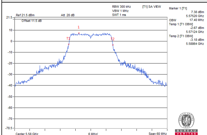
802.11a : CH 116
