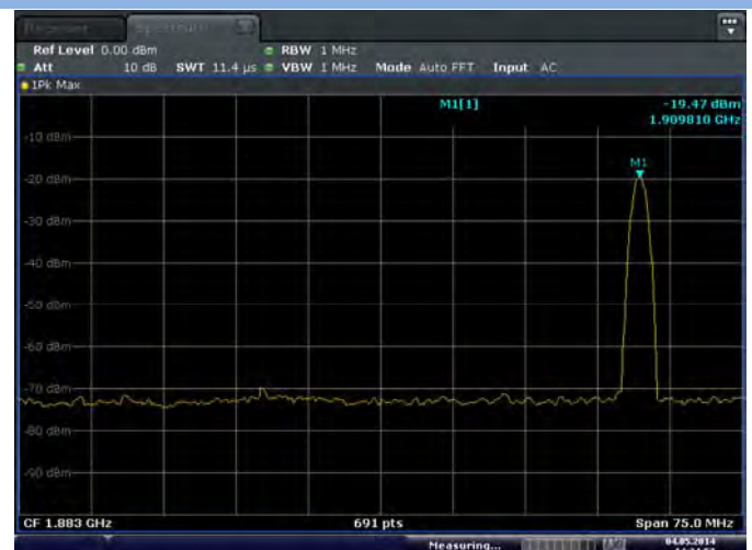
GSM 1900MHz CHANNEL 810
