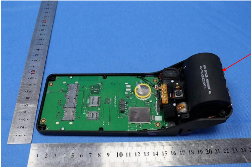
WWAN antenna
