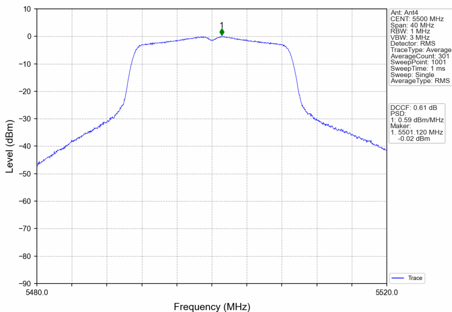
802.11ac(VHT20)_LCH_5500MHz_Ant4_NTNV
